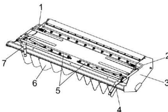
Рисунок 2.17 – Установка дефлектора
