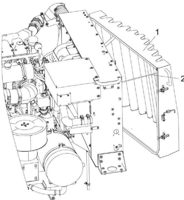
1 – экран воздухозаборника; 2 – упор
