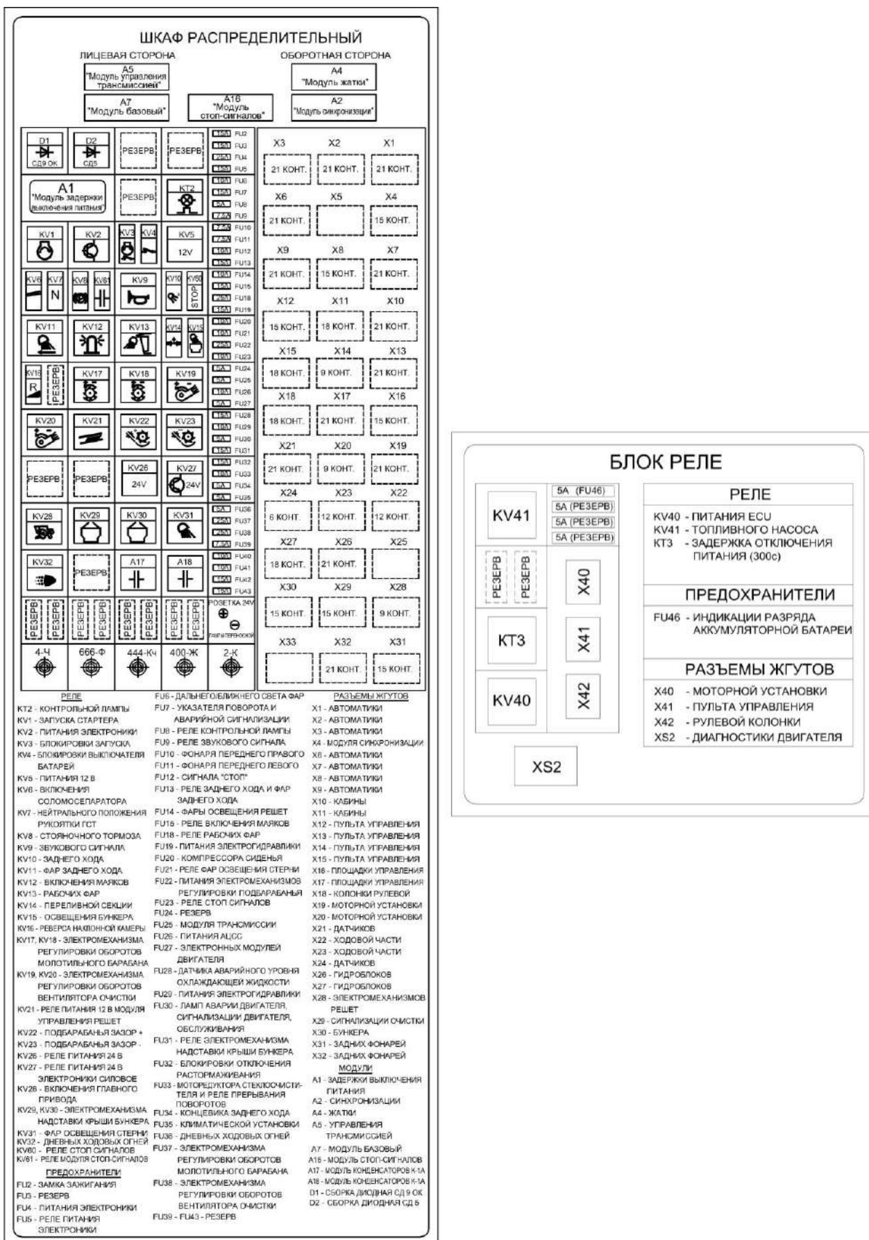
Рисунок 1.24 – Схема соединений шкафа распределительного и блока реле
