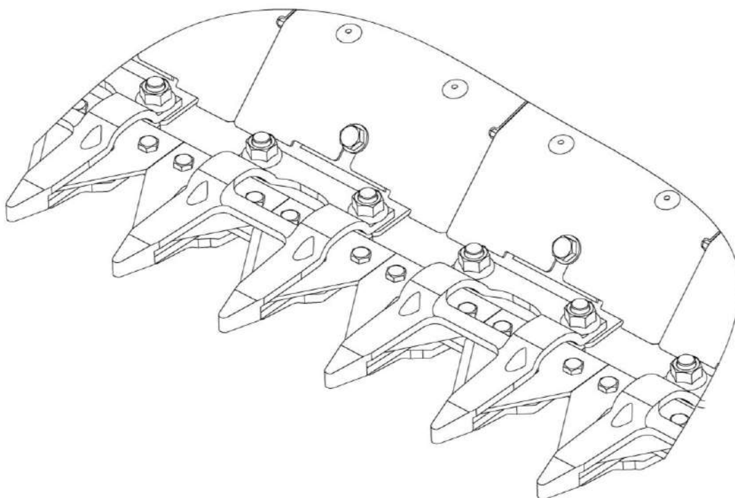
Рисунок 2.1 – Режущий аппарат
