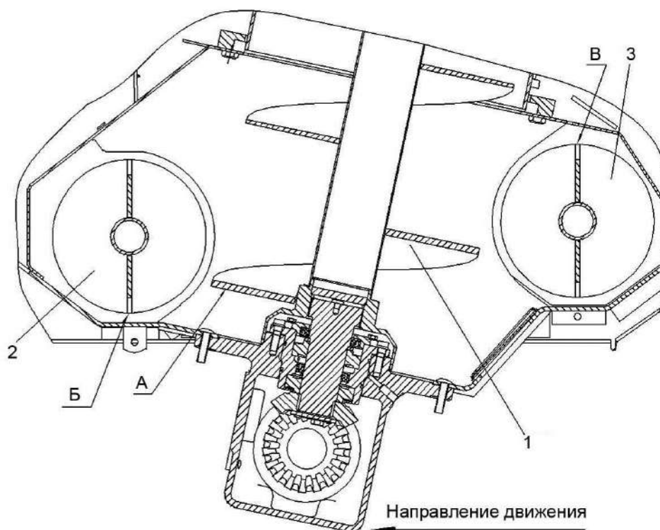
Рисунок 2.38 – Регулировка шнеков выгрузки
