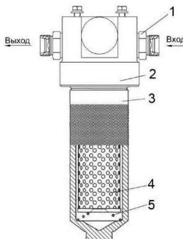
Рисунок 3.5 – Фильтр напорный
