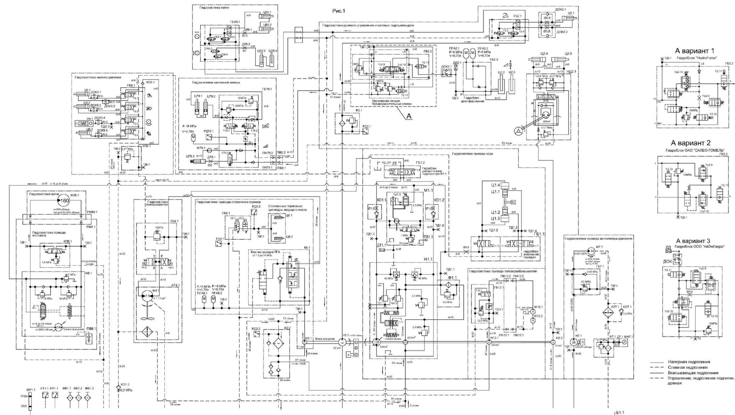
Рисунок А.1 – Схема гидравлическая принципиальная гидросистемы комбайна
