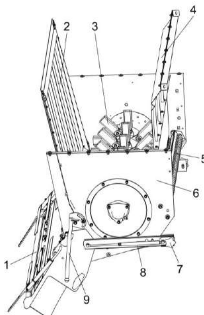
1 – дефлектор; 2 – заслонка; 3 – ротор измельчителя; 4 – стенка; 5 – ножевая опора; 6 – корпус измельчителя; 7 – фиксатор; 8 – ползцы; 9 – рукоятка сектора
