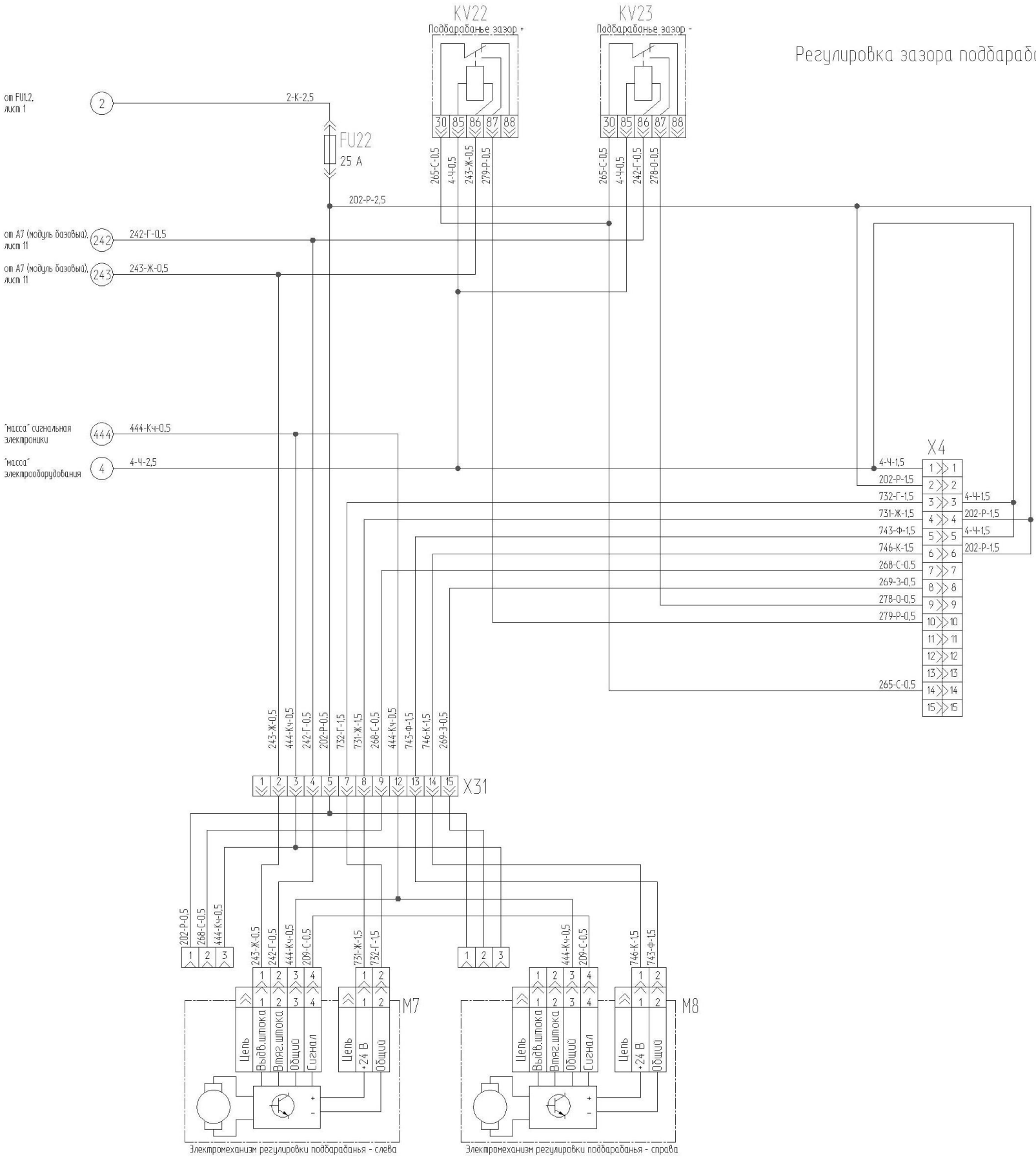
Рисунок Б.13 – Схема электрическая принципиальная комбайна
