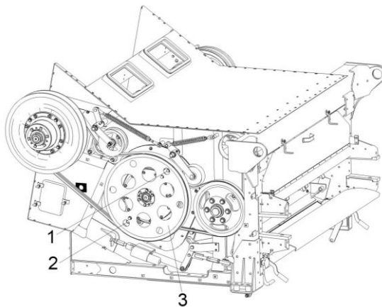
Рисунок 2.19 - Включение редуктора понижения оборотов молотильного барабана
