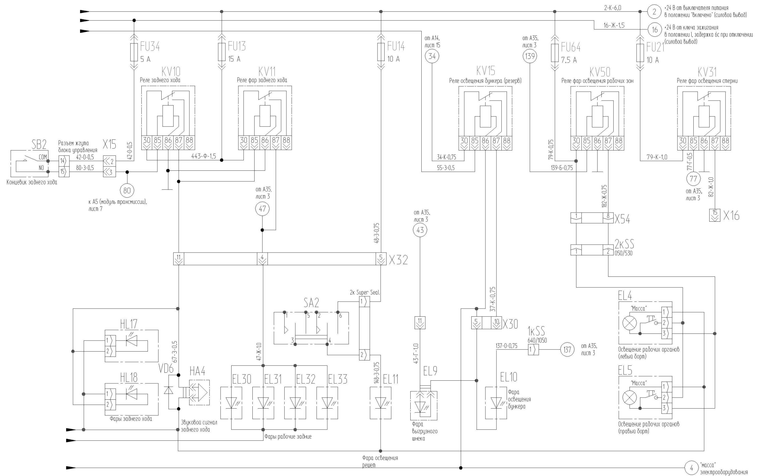
Рисунок Б.2 – Схема электрическая принципиальная комбайна (лист 3)
