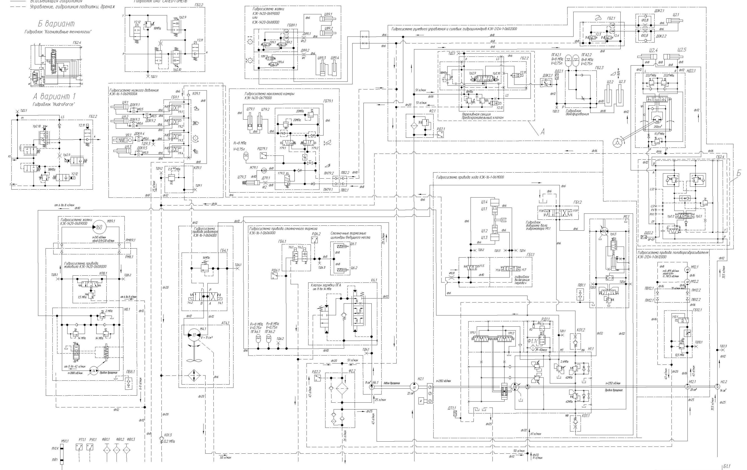
Рисунок А.1 – Схема гидравлическая принципиальная гидросистемы комбайна
