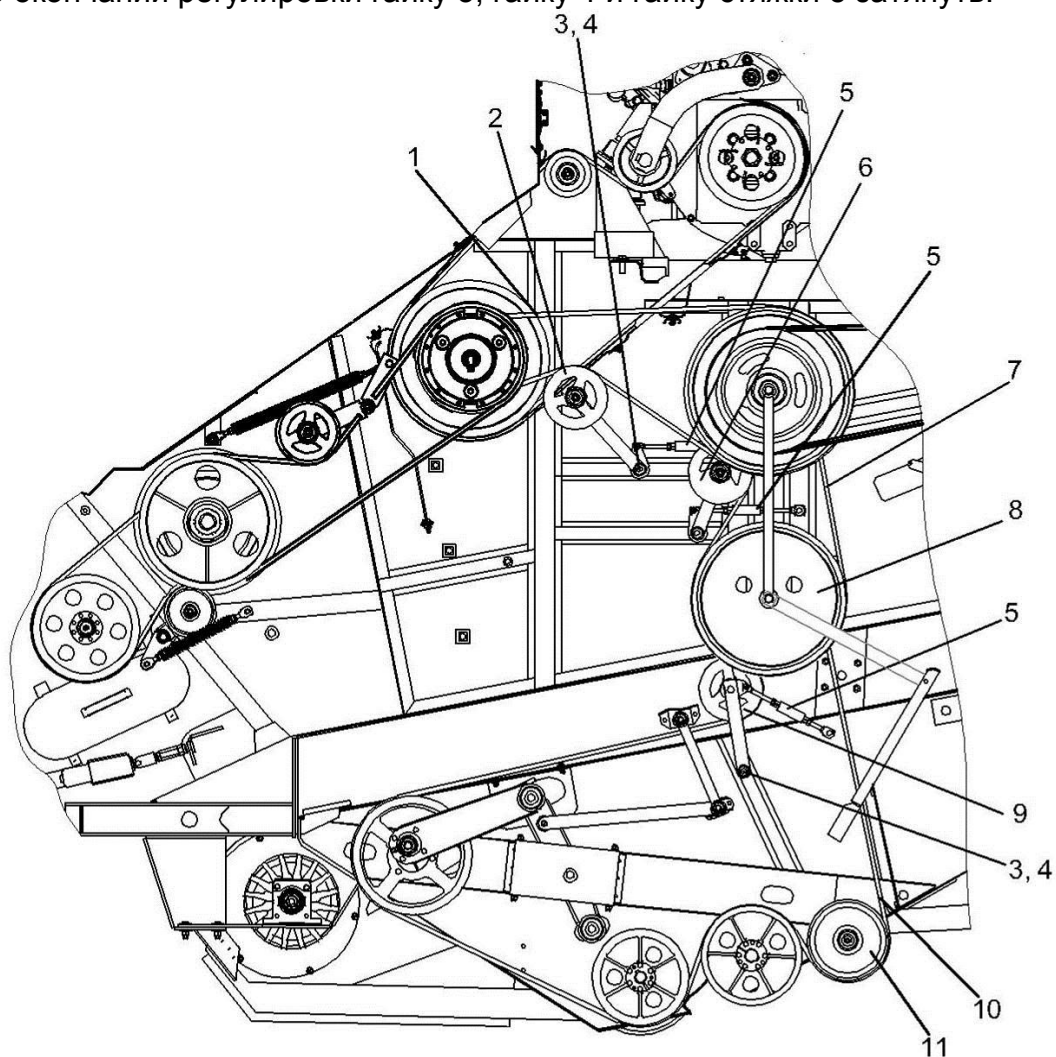
Рисунок 2.23 – Регулировка привода очистки
