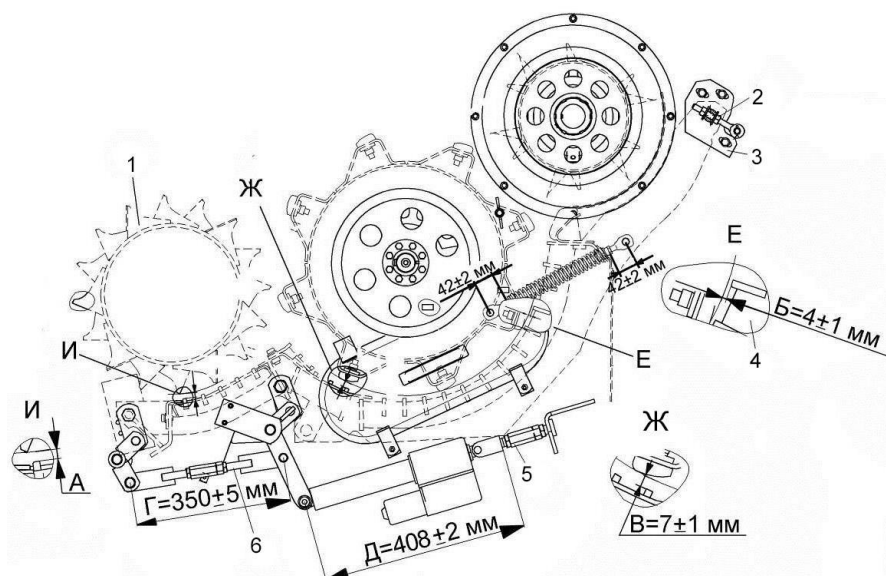
Рисунок 2.18 – Регулировка молотильного аппарата
