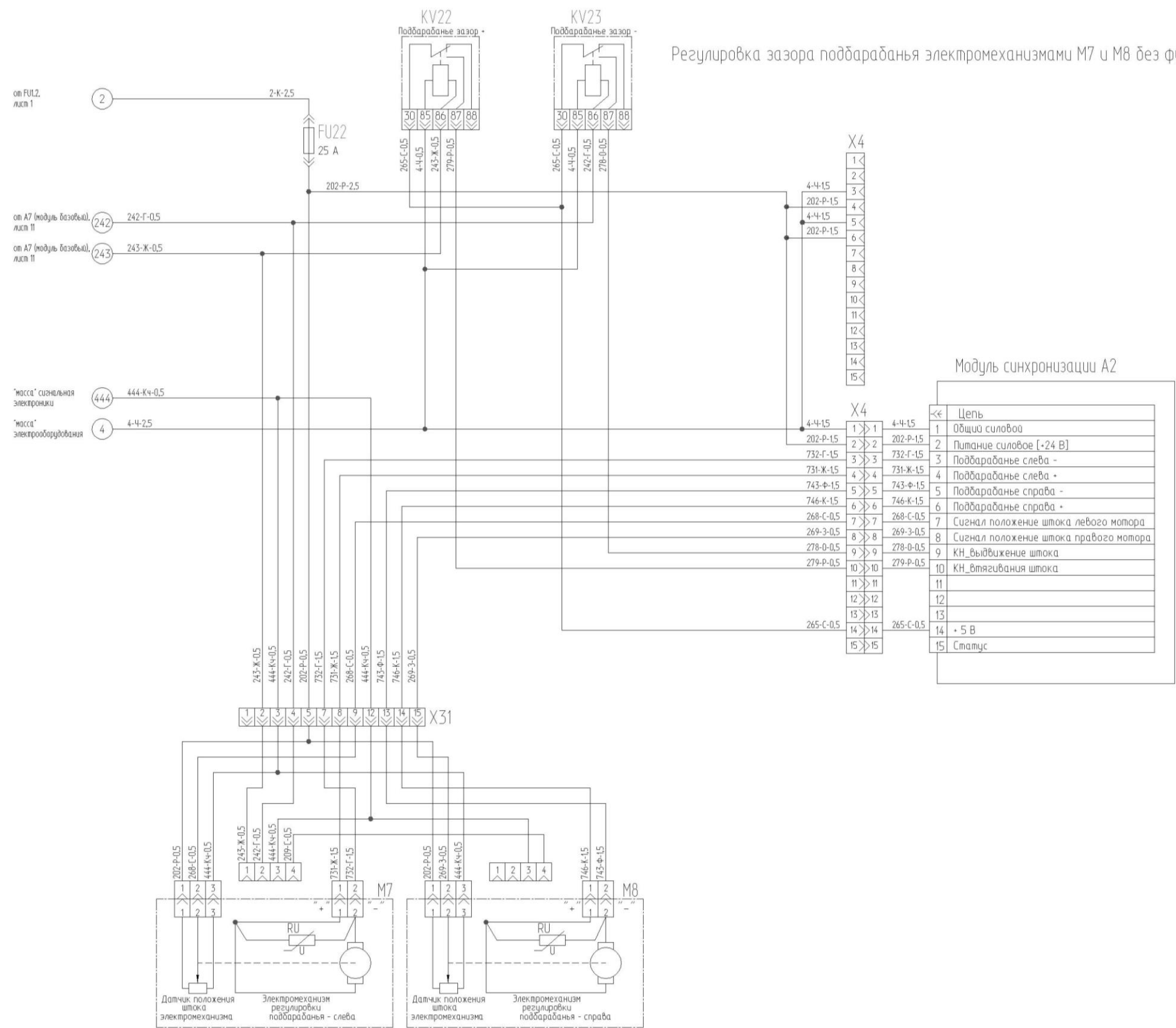
Рисунок Б.12 – Схема электрическая принципиальная комбайна
