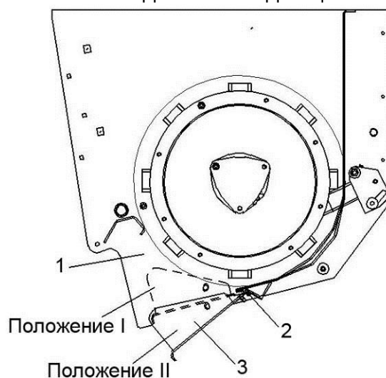
Рисунок 2.24 - Регулировка днища соломоизмельчителя
