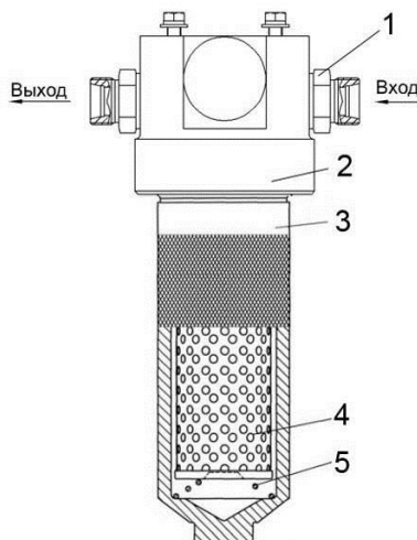
Рисунок 3.5 – Фильтр напорный
