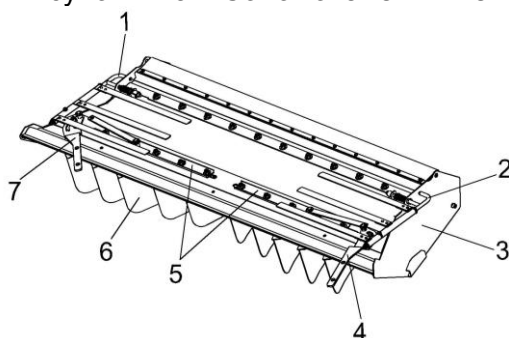
Рисунок 2.16 – Соломоизмельчитель
