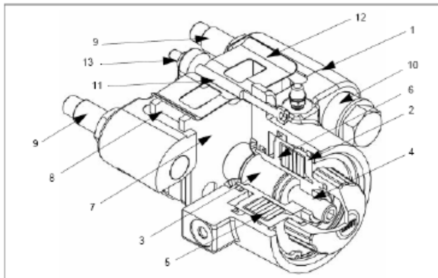
Рисунок 1-1: Компоненты тормоза
