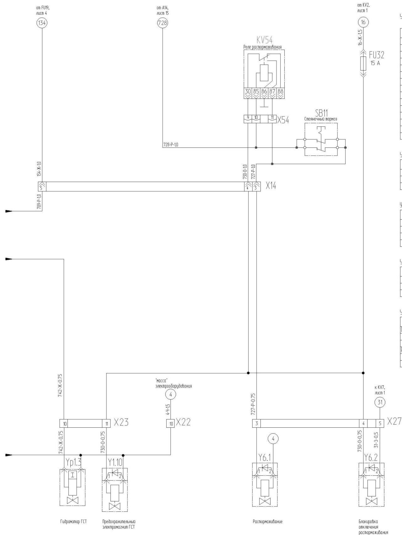
Рисунок Б.7 – Схема электрическая принципиальная комбайна (лист 2)
