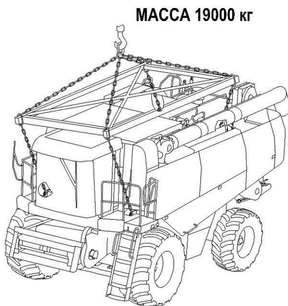
Рисунок 6.1 – Схема строповки комбайна
