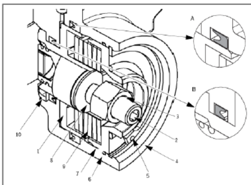
Рисунок 4-3: Замена уплотнений
