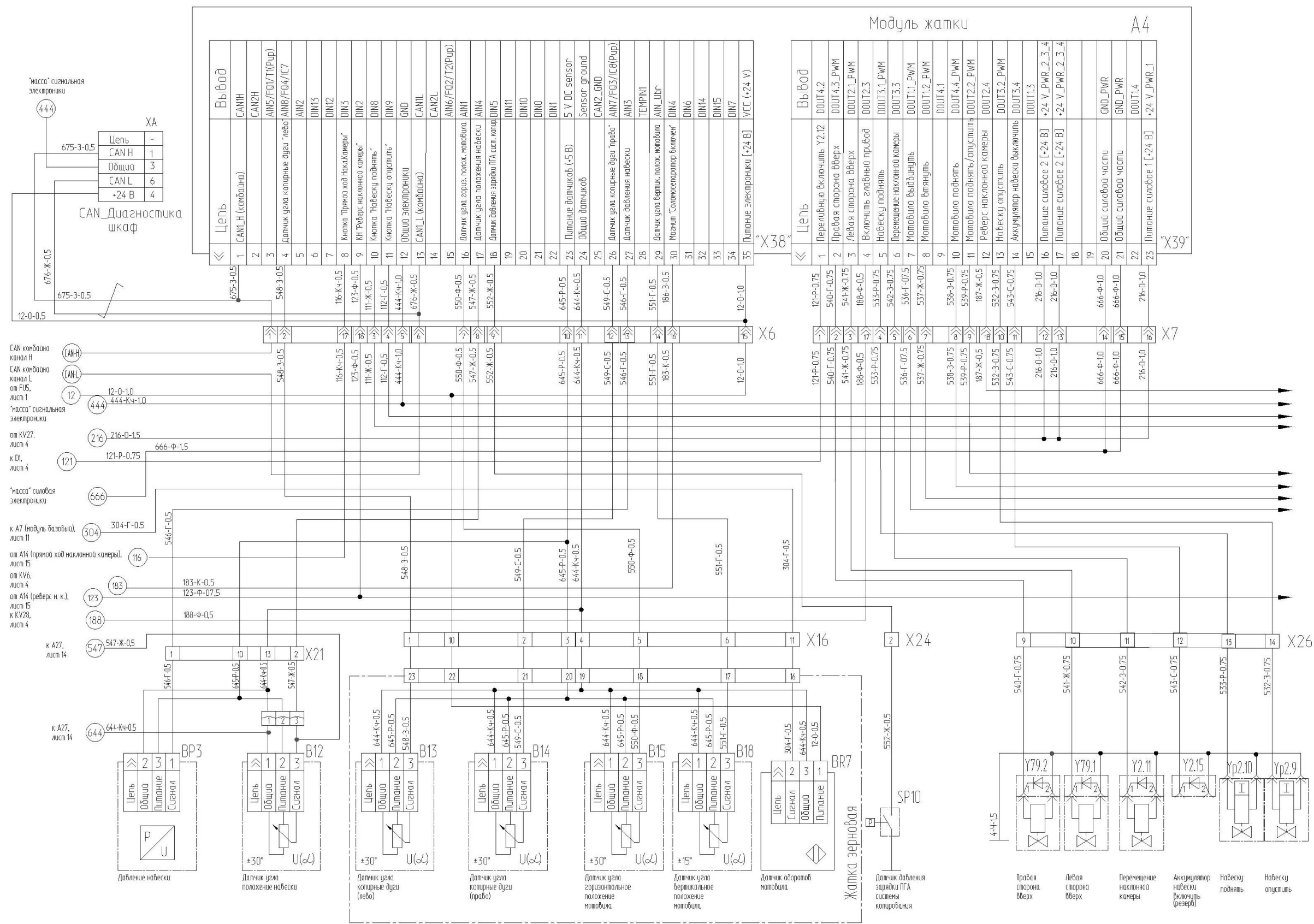
Рисунок Б.9 – Схема электрическая принципиальная комбайна (лист 1)
