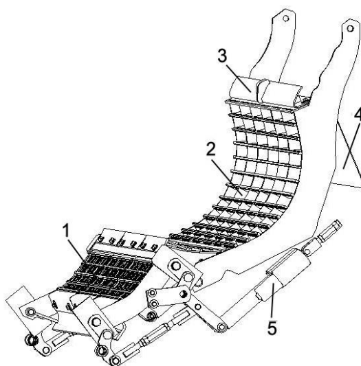
1 – переднее подбарабанье; 2 – заднее подбарабанье; 3 – козырек; 4 – фартук; 5 – механизм подъема подбарабаний
