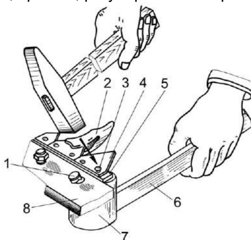
1 – штырь; 2 – палец; 3 – заклепка; 4 – сегмент; 5 – спинка ножевая; 6 – рукоятка; 7 – корпус; 8 – брус пальцевый
