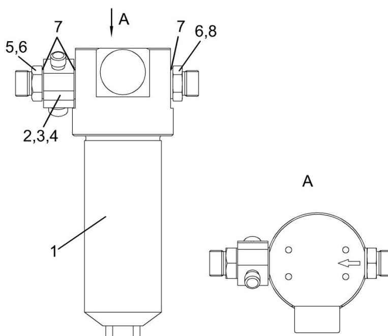
Рисунок 1.20 – Фильтр сливной
