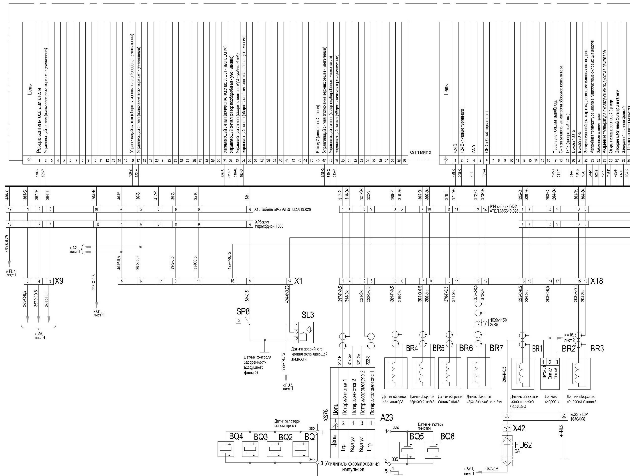
Рисунок Б.6 – Схема электрическая принципиальная комбайна (лист 6.1)
