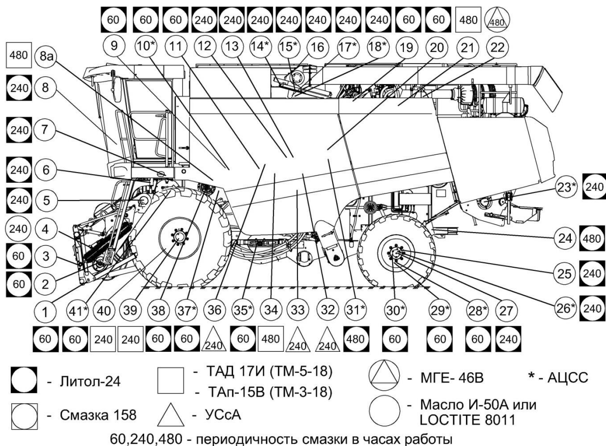
Рисунок 3.5 – Смазка комбайна (вид слева)
