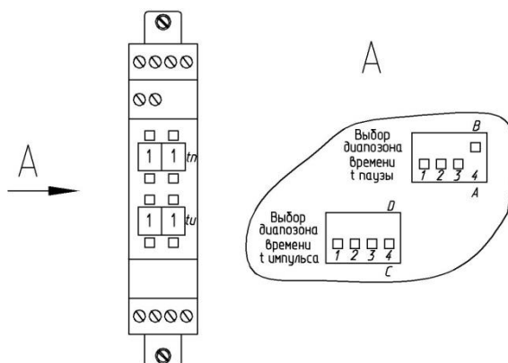
Рисунок 1.36 – Реле времени
