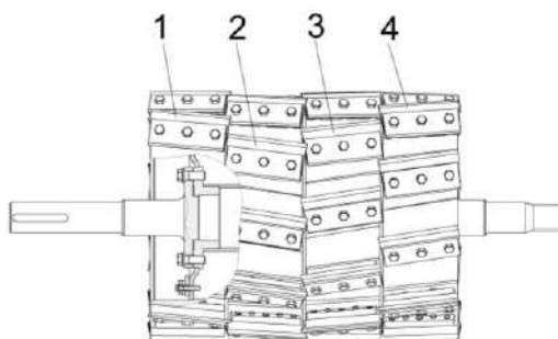
1,2,3,4 – ножи
