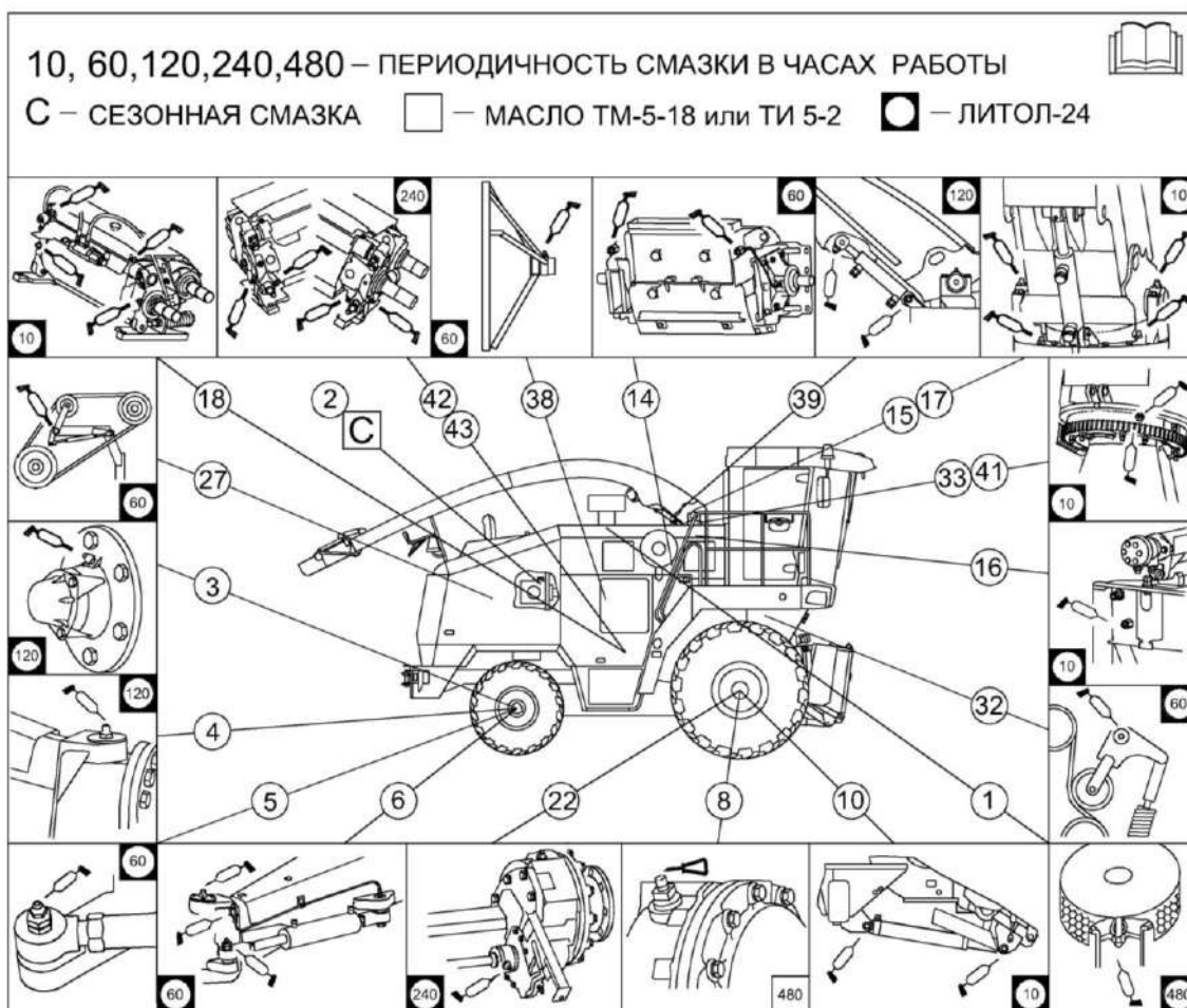
Рисунок 3.12 – Схема смазки комбайна (вид справа)
