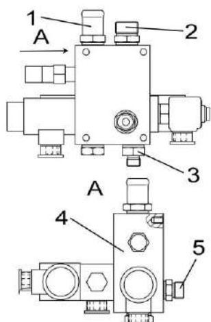
Рисунок 1.9 – Гидроблок навески ГБ1
