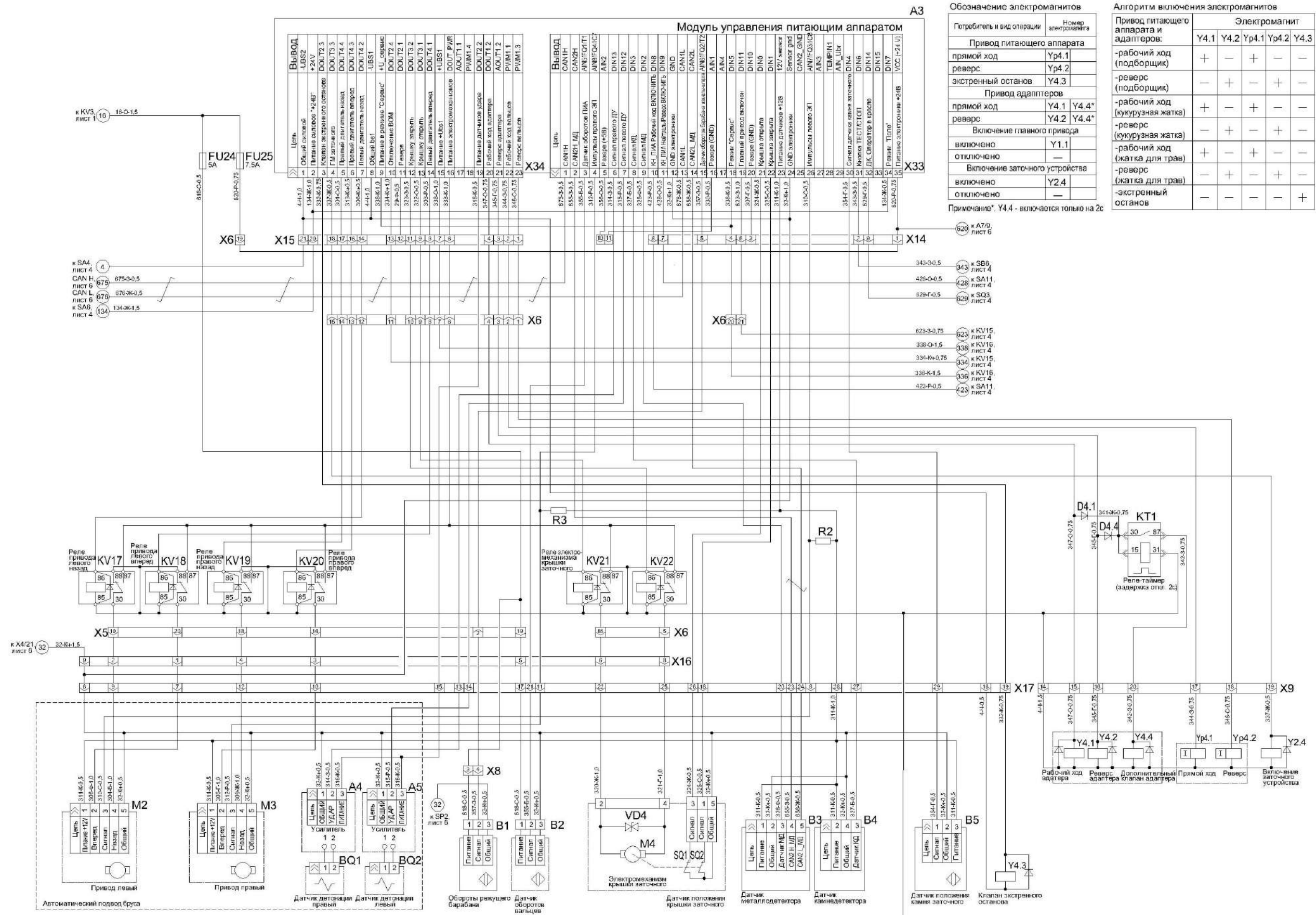
Рисунок Б.5 – Схема электрическая принципиальная комбайна
