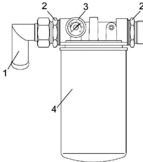
Рисунок 1.12 – Фильтр сливной
