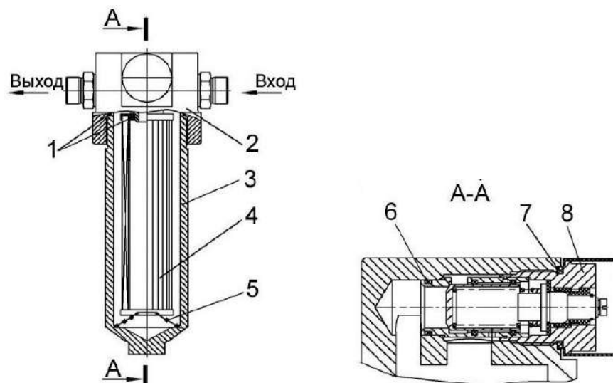
Рисунок 1.12 – Фильтр сливной
