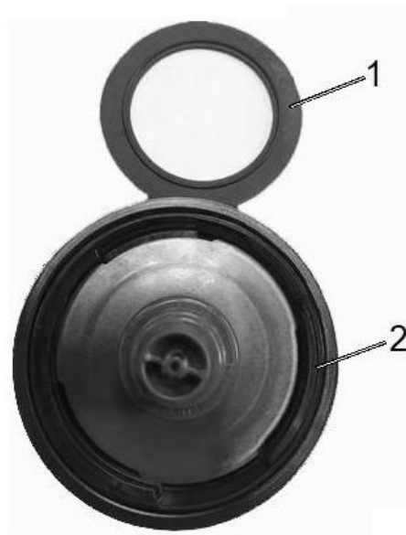
Рисунок 2 - Извлечение прокладки
