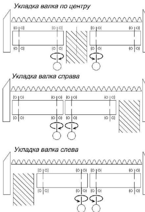
Рисунок 1.6 - Схема укладки валков
