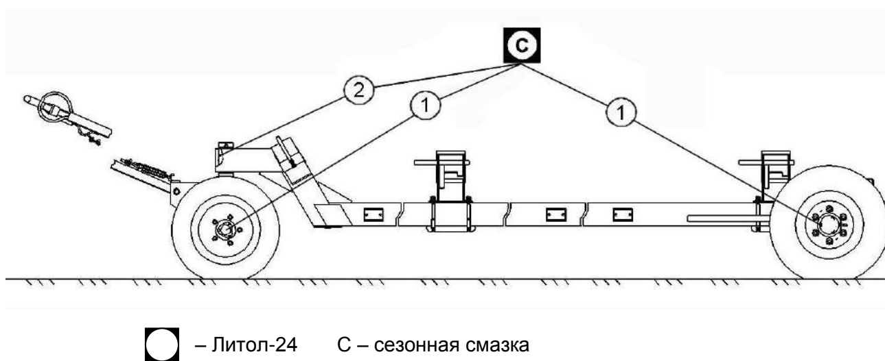
Рисунок 3.2 – Схема смазки транспортной тележки
