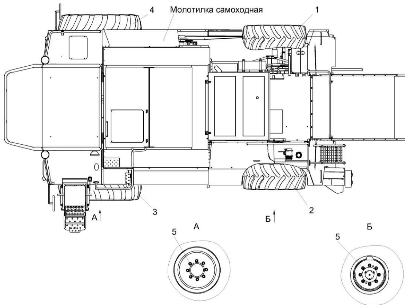
Рисунок 111 – Установка колес КЗК-8К-0111100
