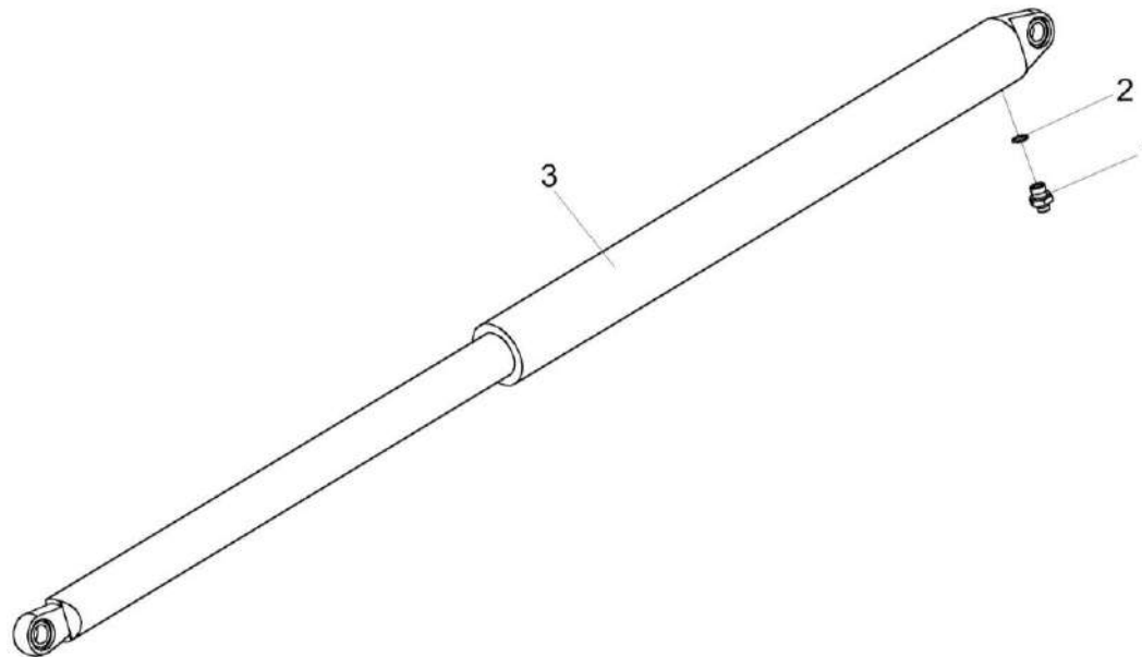
Рисунок 273– Гидроцилиндр КЗК-8-8-0602510
