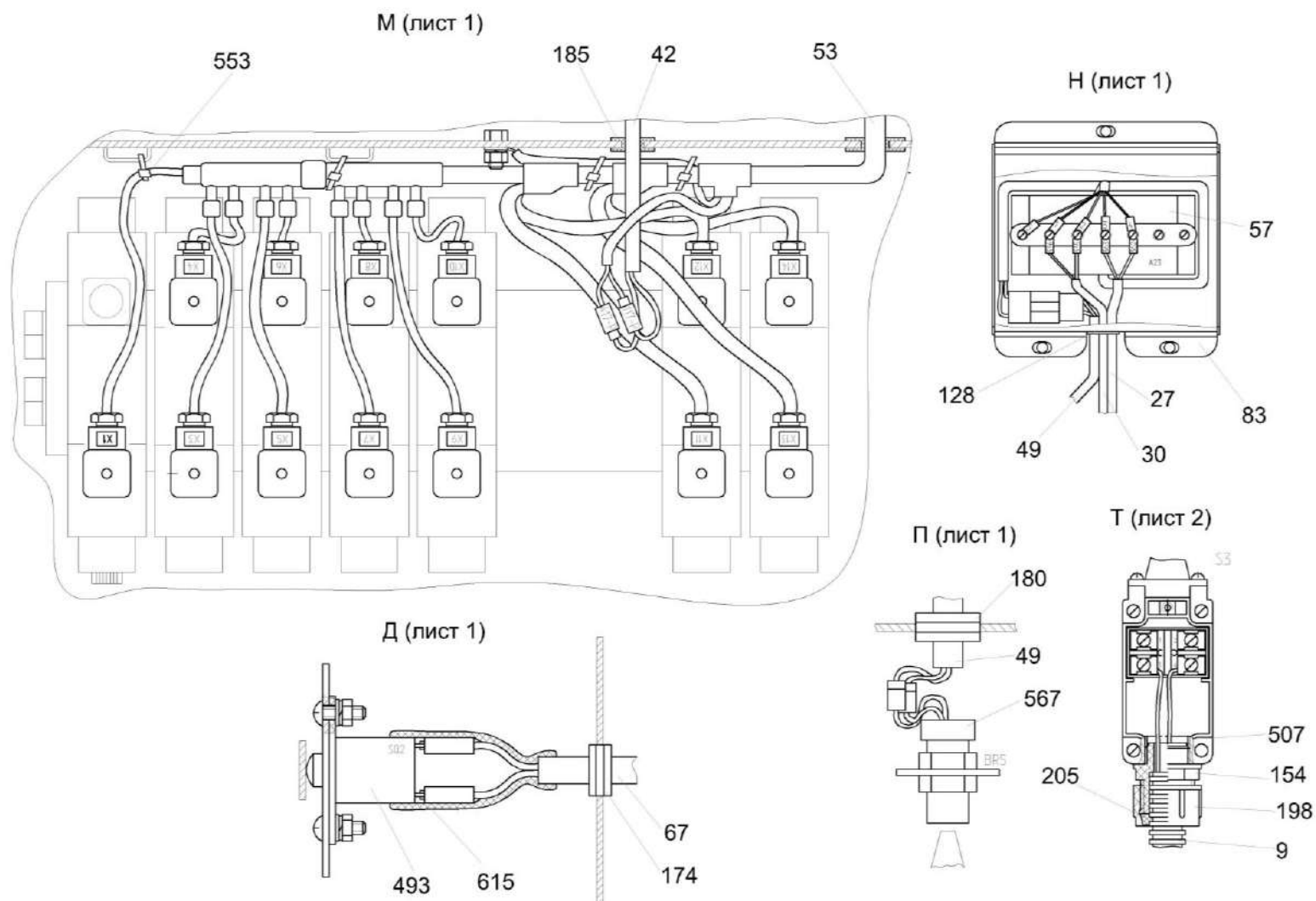
Рисунок 243 - Установка электрооборудования молотилки КЗК-400-2-0721000 (лист 5)
