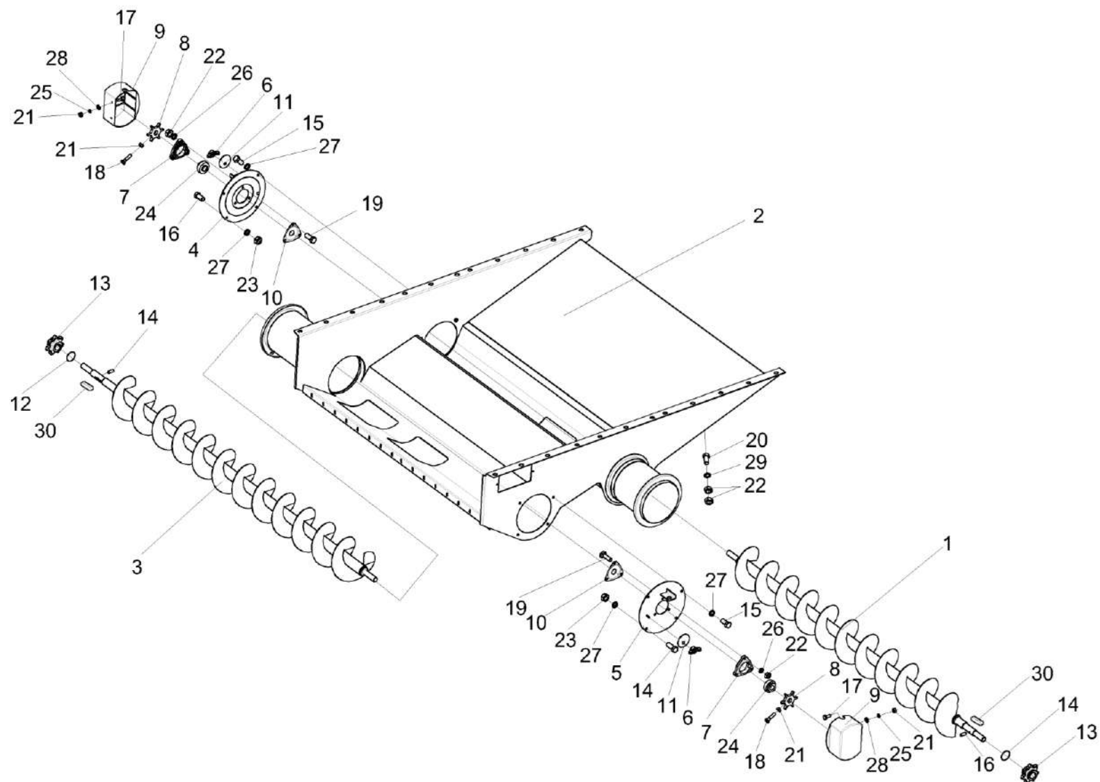
Рисунок 27 – Блок шнеков КЗК 0218010Г
