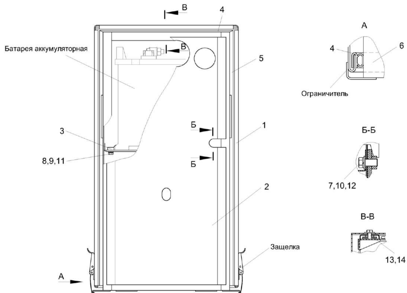
Рисунок 218 – Ящик аккумуляторный КЗК-12-0129000А
