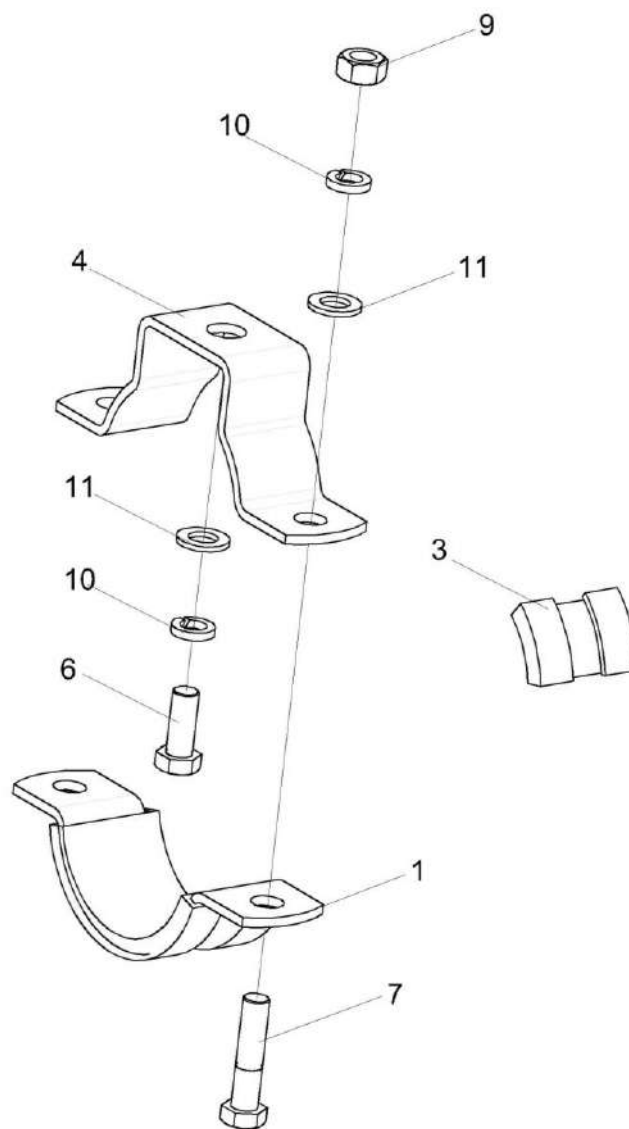
Рисунок 159 – Установка ресивера КЗК-8-3-0113050
