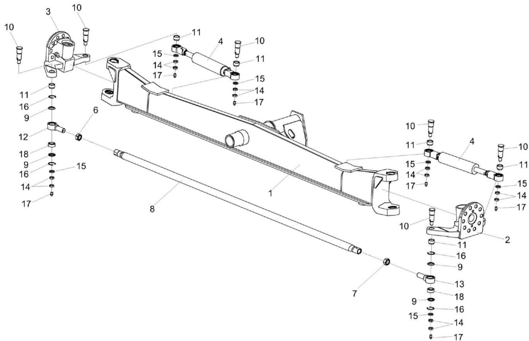
Рисунок 45 – Мост управляемых колёс КЗК-8К-0109000 (лист 2)
