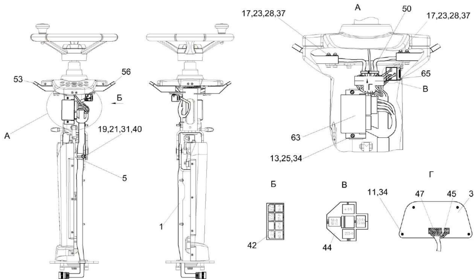
Рисунок 246 - Установка электрооборудования колонки рулевой КЗК-400-2-0723000
