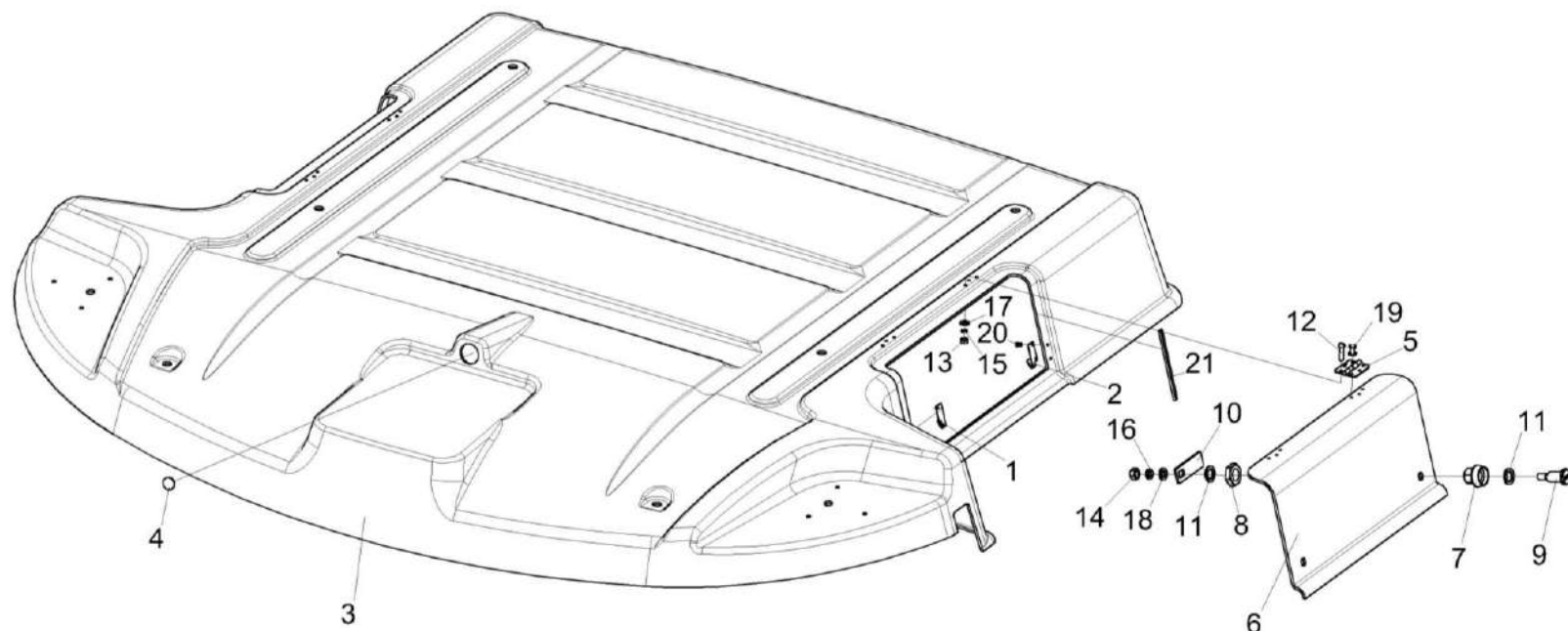
Рисунок 149 – Крыша УКЗ-01-0101230
