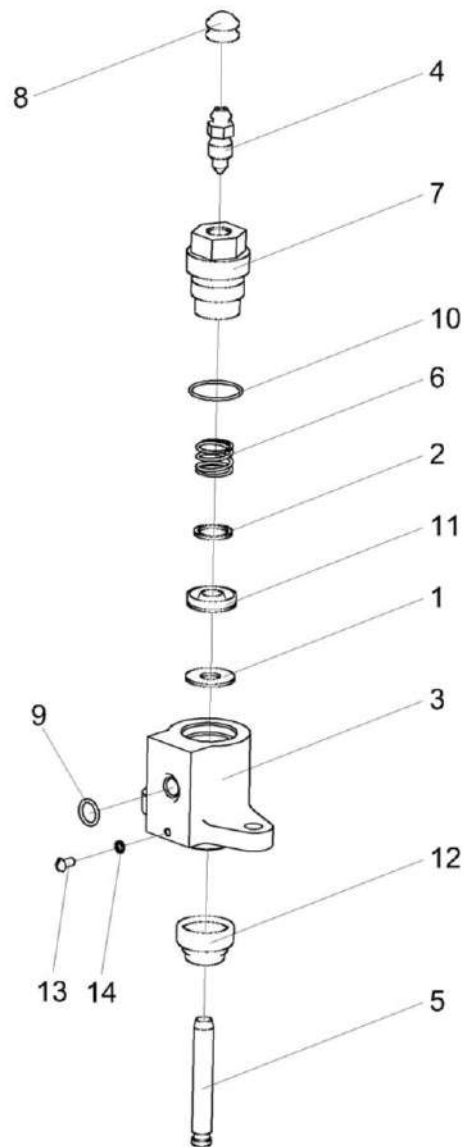
Рисунок 42 – Гидроцилиндр КЗК-12-0107200-01
