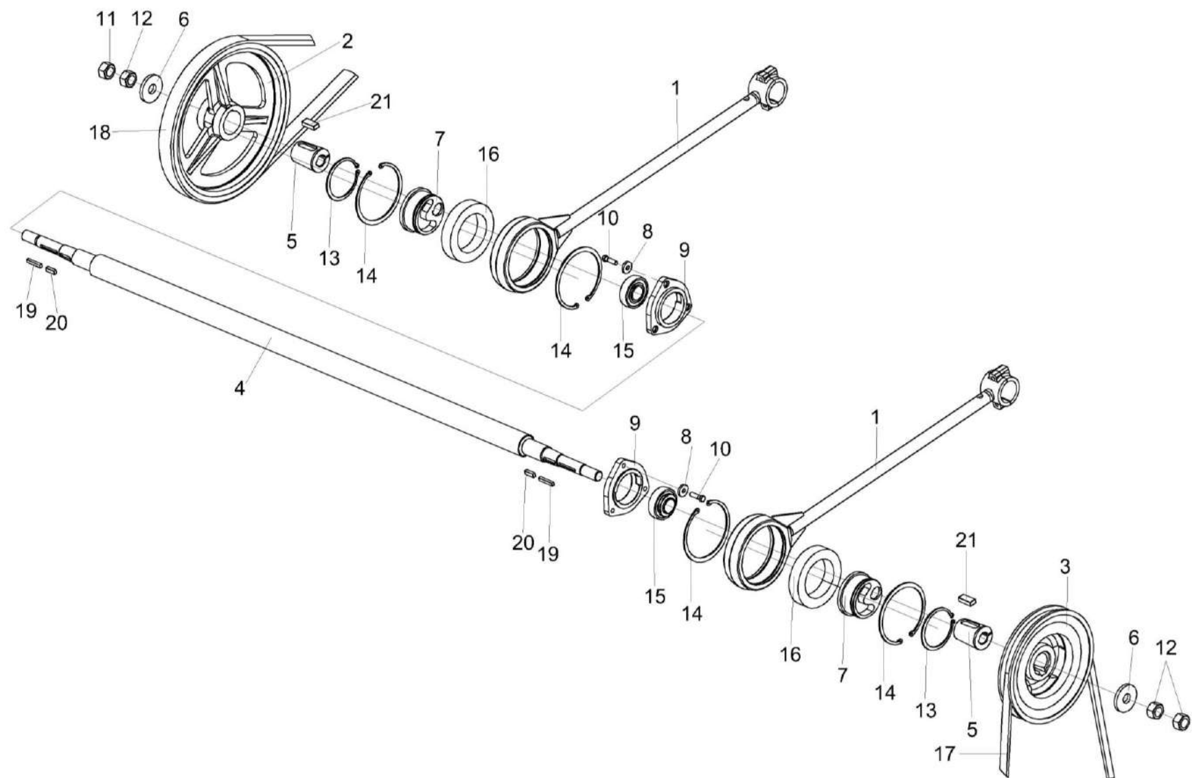
Рисунок 70 – Установка шатуна КЗР 0202030Е и шкивов КЗК-5-4-0202120, КЗК-8А-0202111
