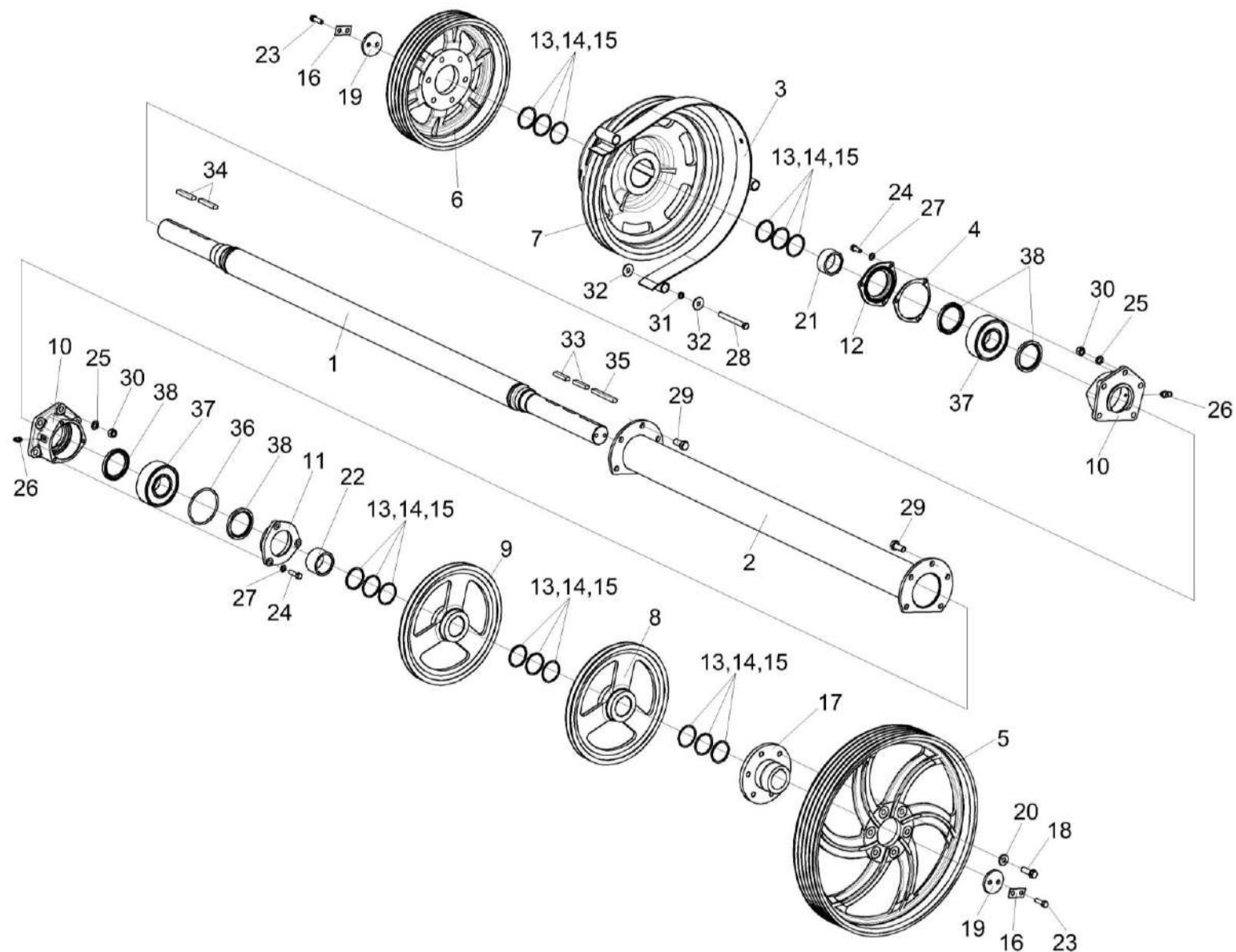
Рисунок 62 – Установка шкивов КЗК 0202860А и КЗК 0202103Б
