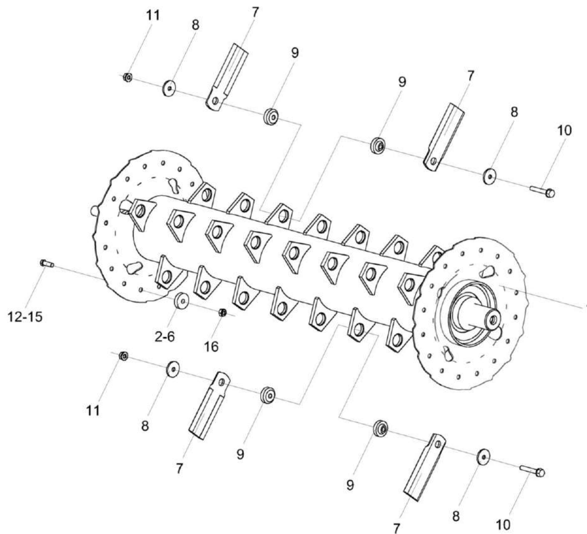
Рисунок 122 - Ротор измельчителя КЗК-8-9-0290140
