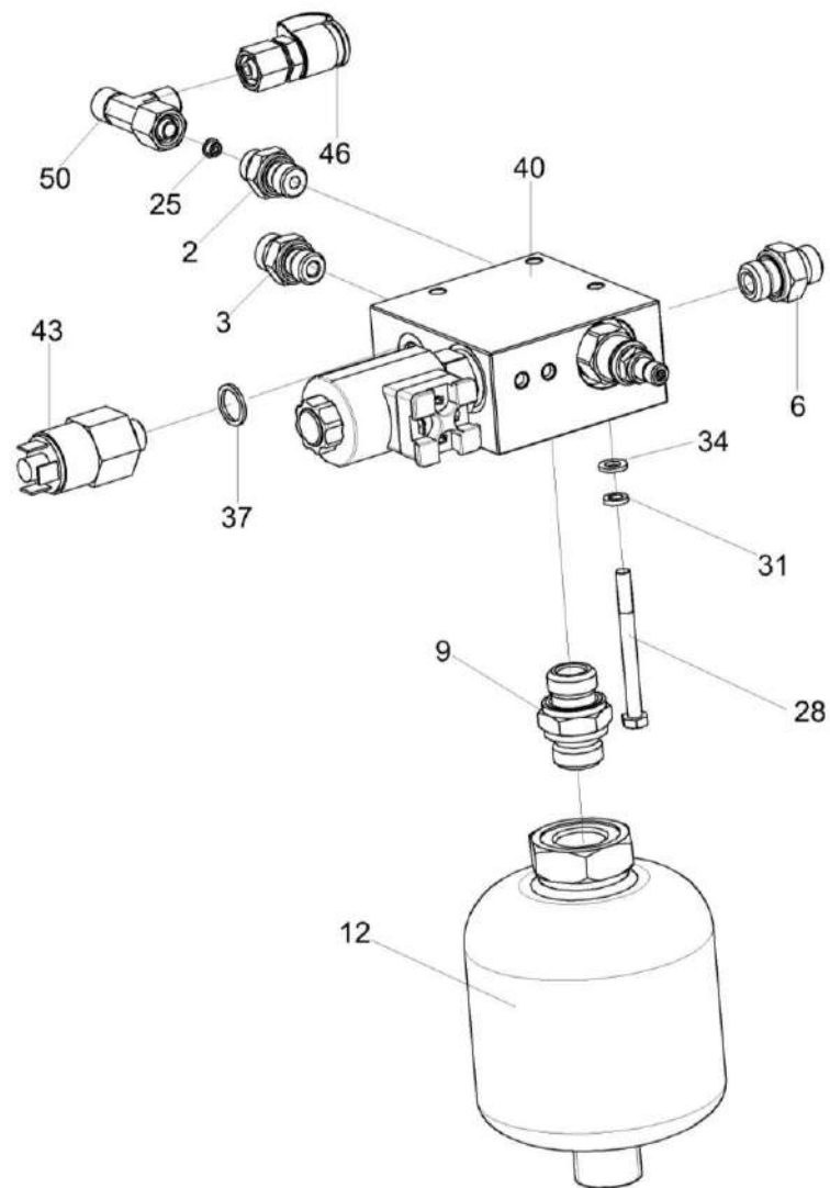
Рисунок 258 - Гидроблок КЗК-400-2-0604300
