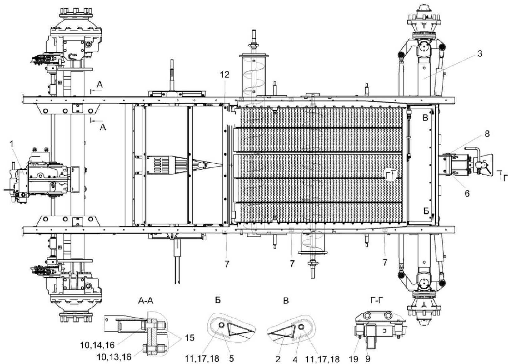
Рисунок 23 - Шасси КЗК-8-9-0111000 (лист 2)
