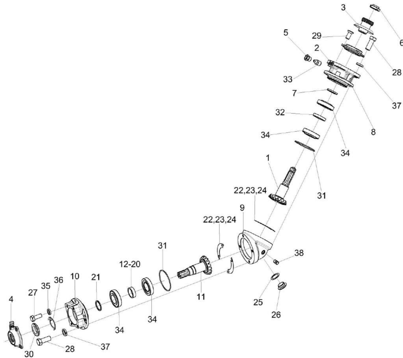
Рисунок 94 – Редуктор КЗК-12-0245500
