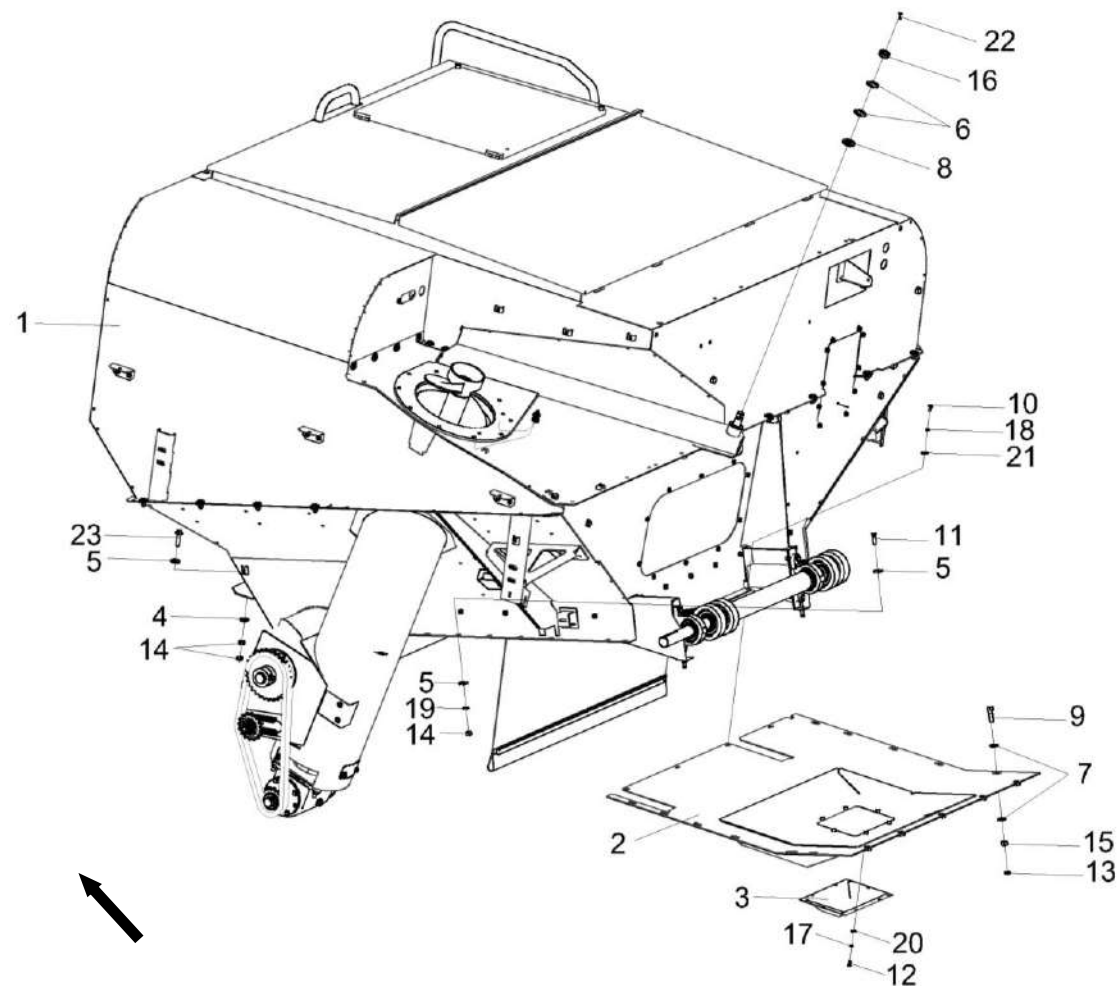
Рисунок 80 - Установка бункера КЗК-8-9-0203000
