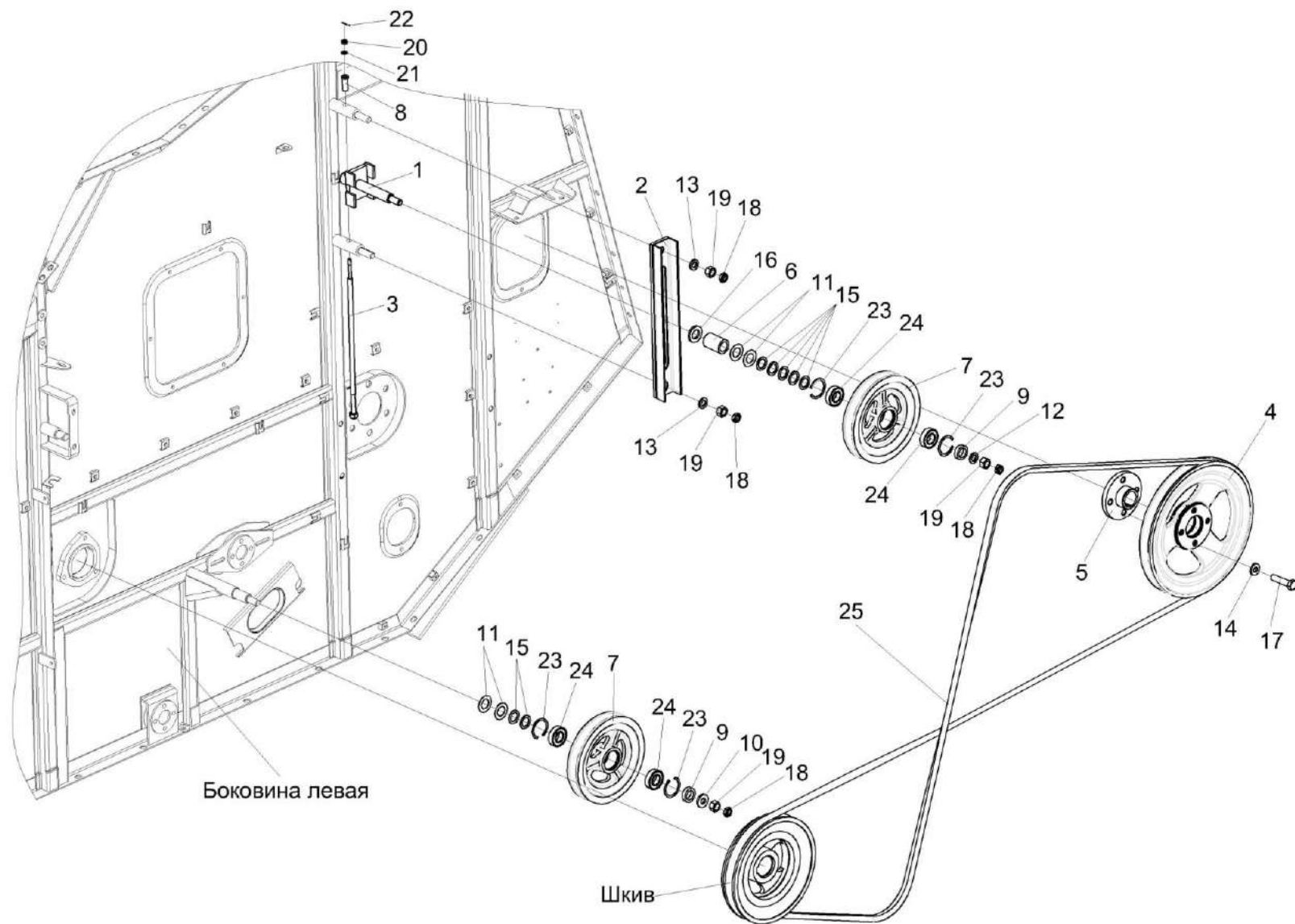
Рисунок 48 – Установка привода солоотряса
