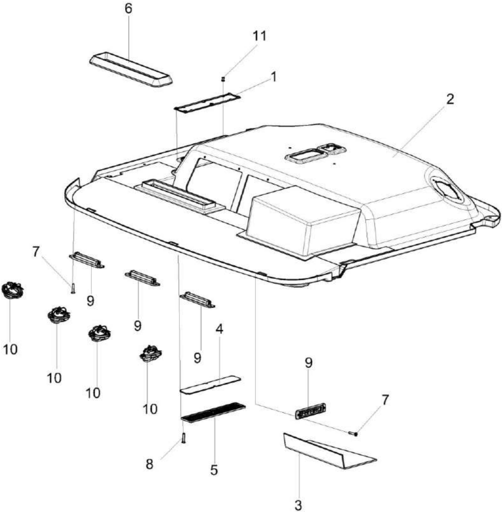
Рисунок 150 – Потолок УКЗ-01-0101280
