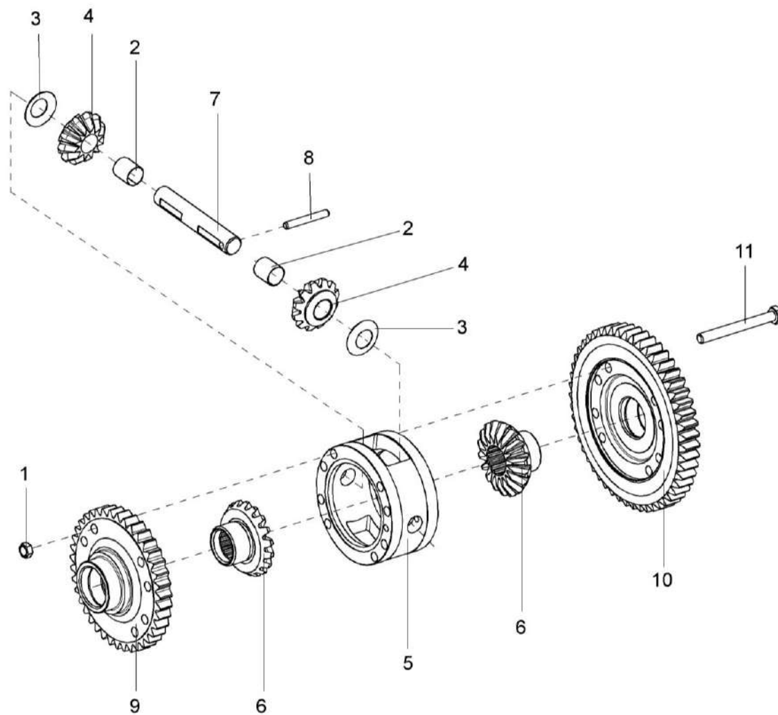
Рисунок 40 – Дифференциал КЗК-8-0107540
