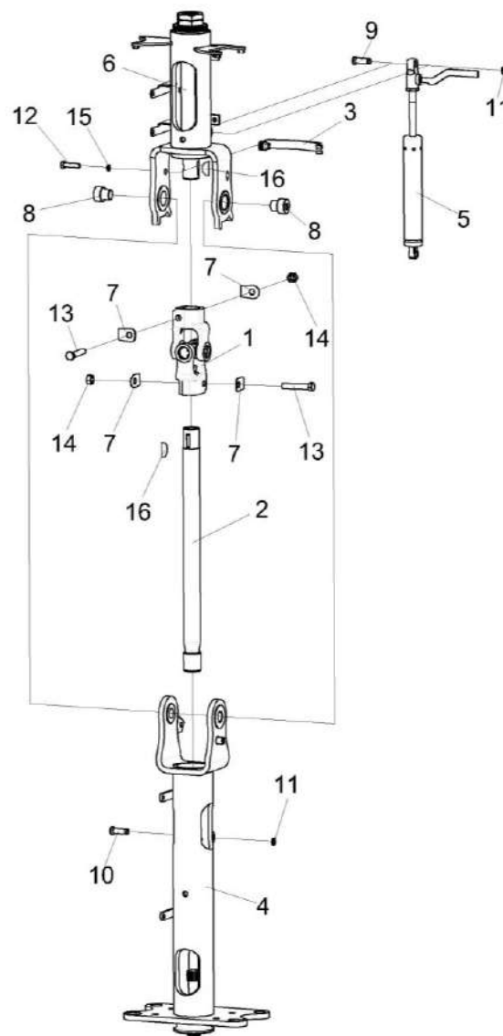
Рисунок 137 – Каркас КЗК-13-0119240
