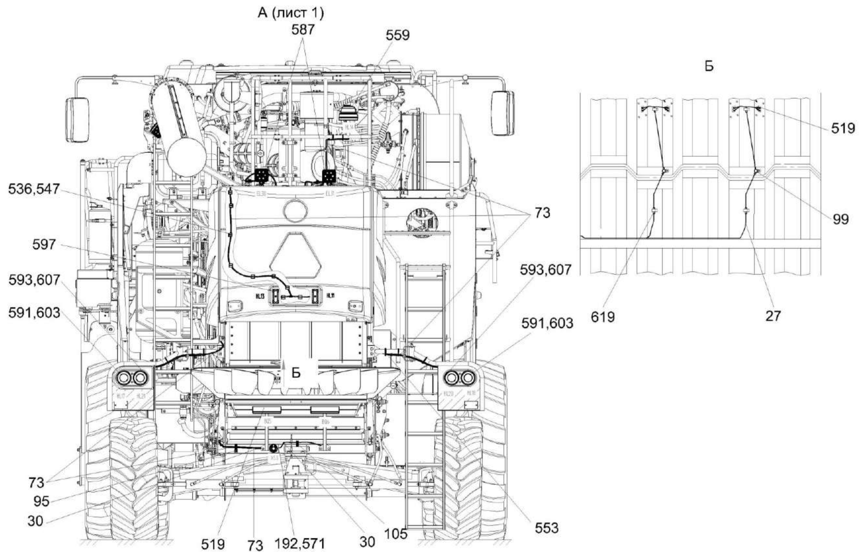
Рисунок 241 - Установка электрооборудования молотилки КЗК-400-2-0721000 (лист 3)
