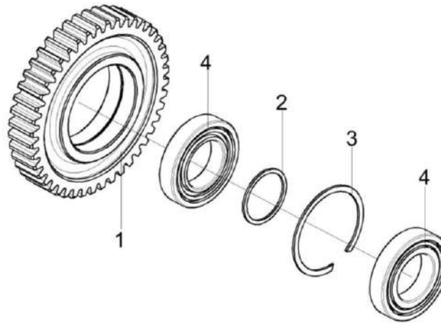
Рисунок 175 – Шестерня КЗК-12-0114010
