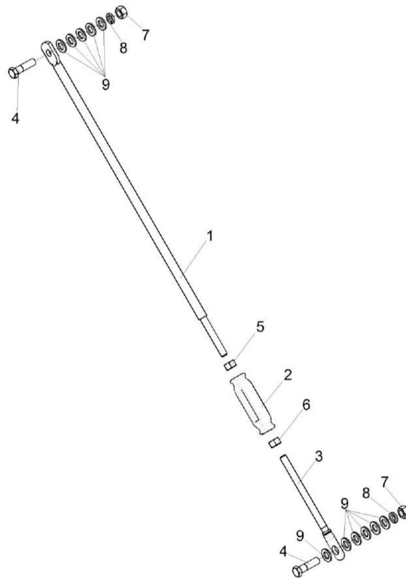
Рисунок 181 – Растяжка КЗК-12-6-0106300
