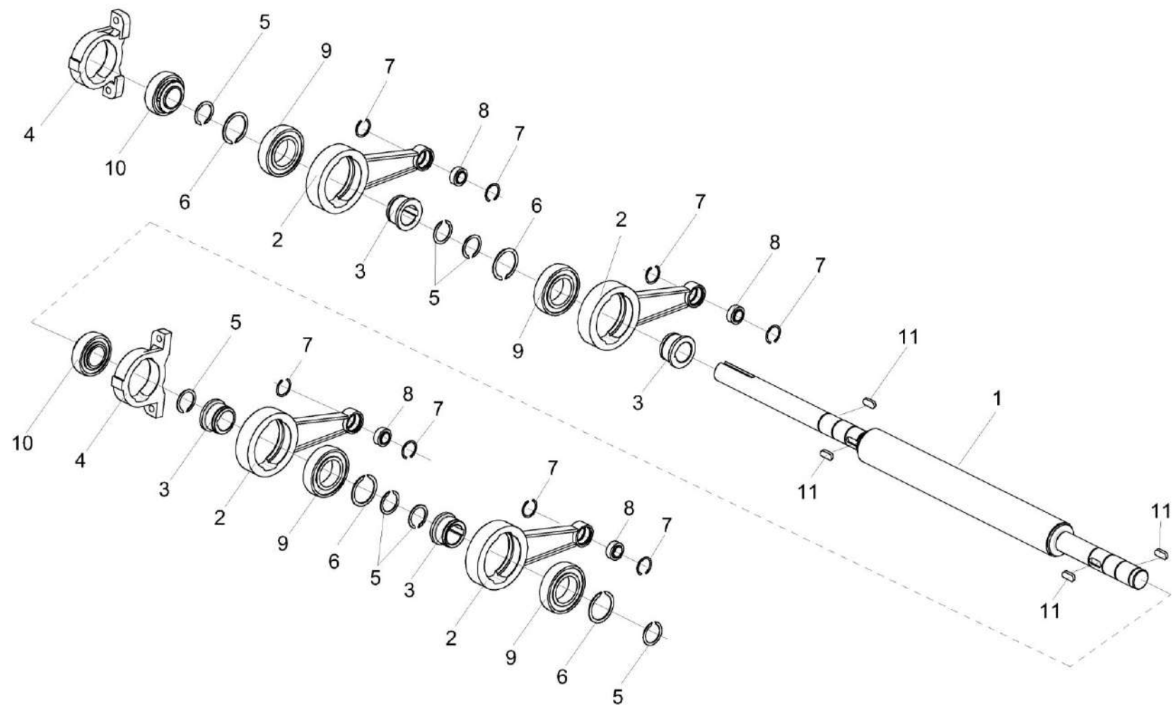
Рисунок 92 – Вибропобудитель КЗК-8-9-0226010
