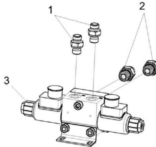
Рисунок 255 - Гидроблок доворота вала ГСТ КЗК-400-2-0601300
