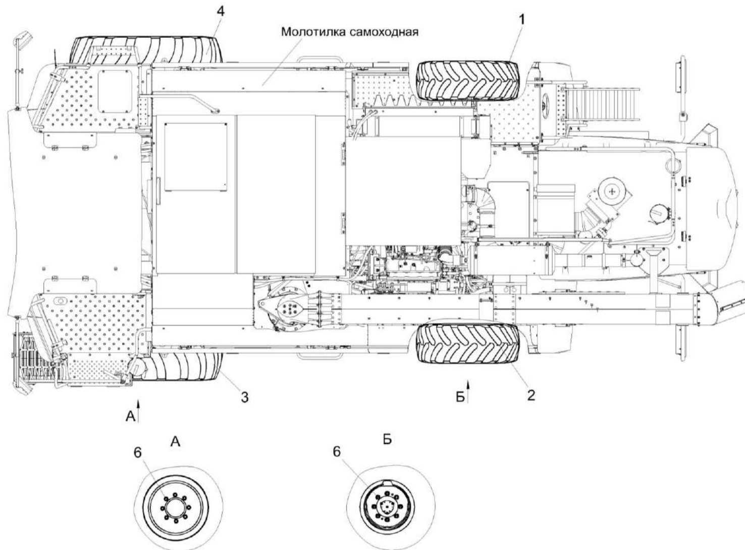
Рисунок 114 – Установка колес КЗК-400-2-0111100
