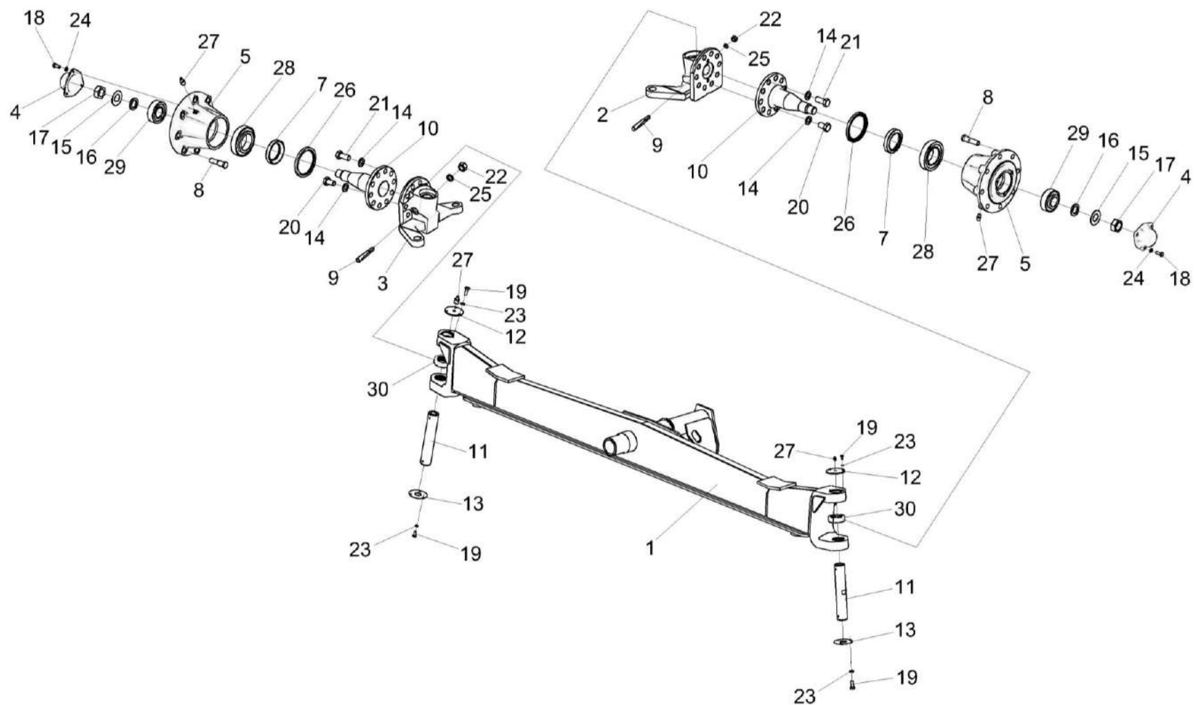
Рисунок 44 – Мост управляемых колёс КЗК-8К-0109000 (лист 1)
