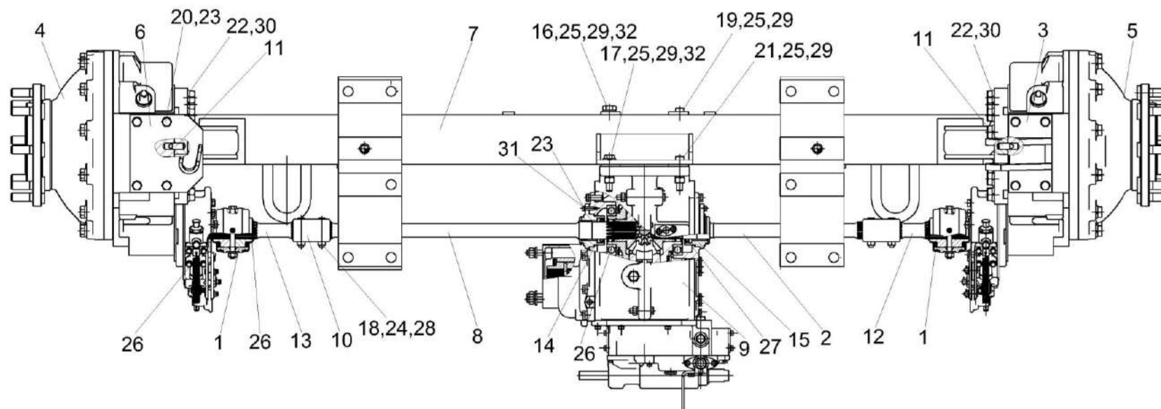
Рисунок 31 – Мост ведущий КЗК-400-1-0107000
