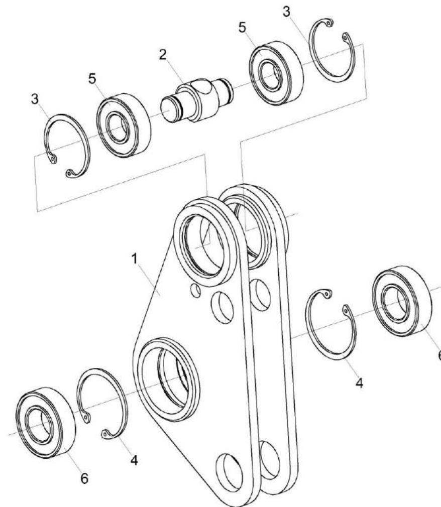
Рисунок 21 – Рычаг КЗК 1785000
