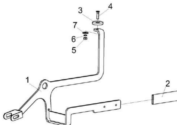
Рисунок 228 – Рукоятка КЗК-400-0121160
