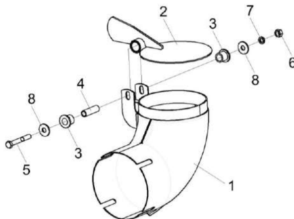
Рисунок 187 – Труба КЗК-12-3-0126880
