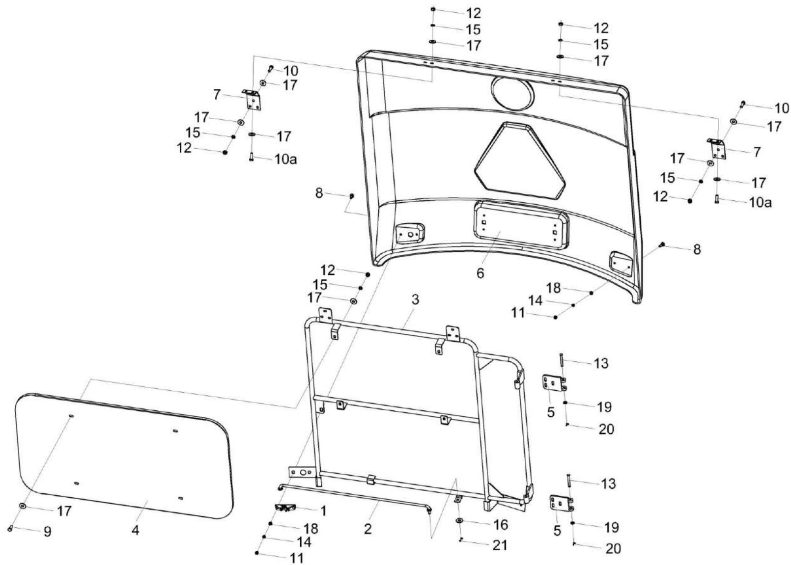
Рисунок 207 – Капот КЗК-8-9-0228020
