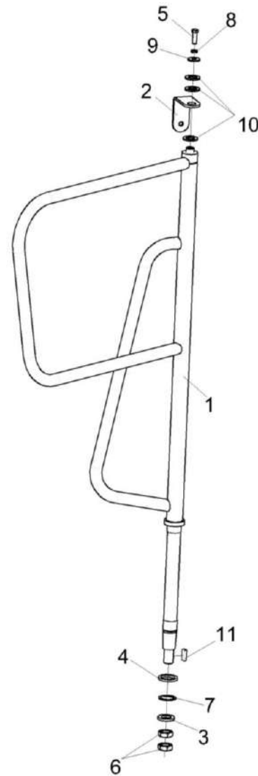
Рисунок 227 – Установка поручня КЗК-8-9-0121060
