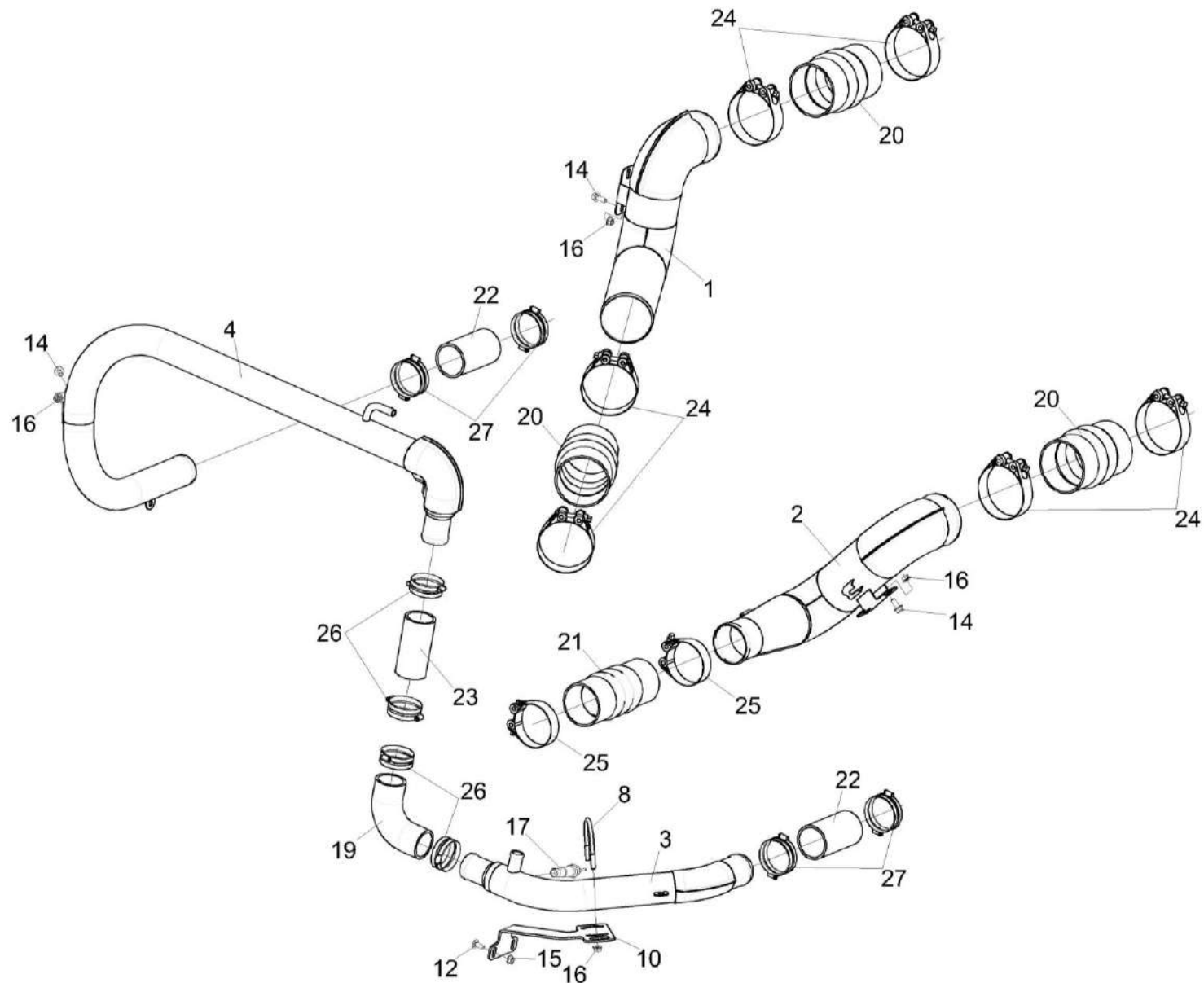
Рисунок 180 – Установка труб КЗК-400-2-0106100
