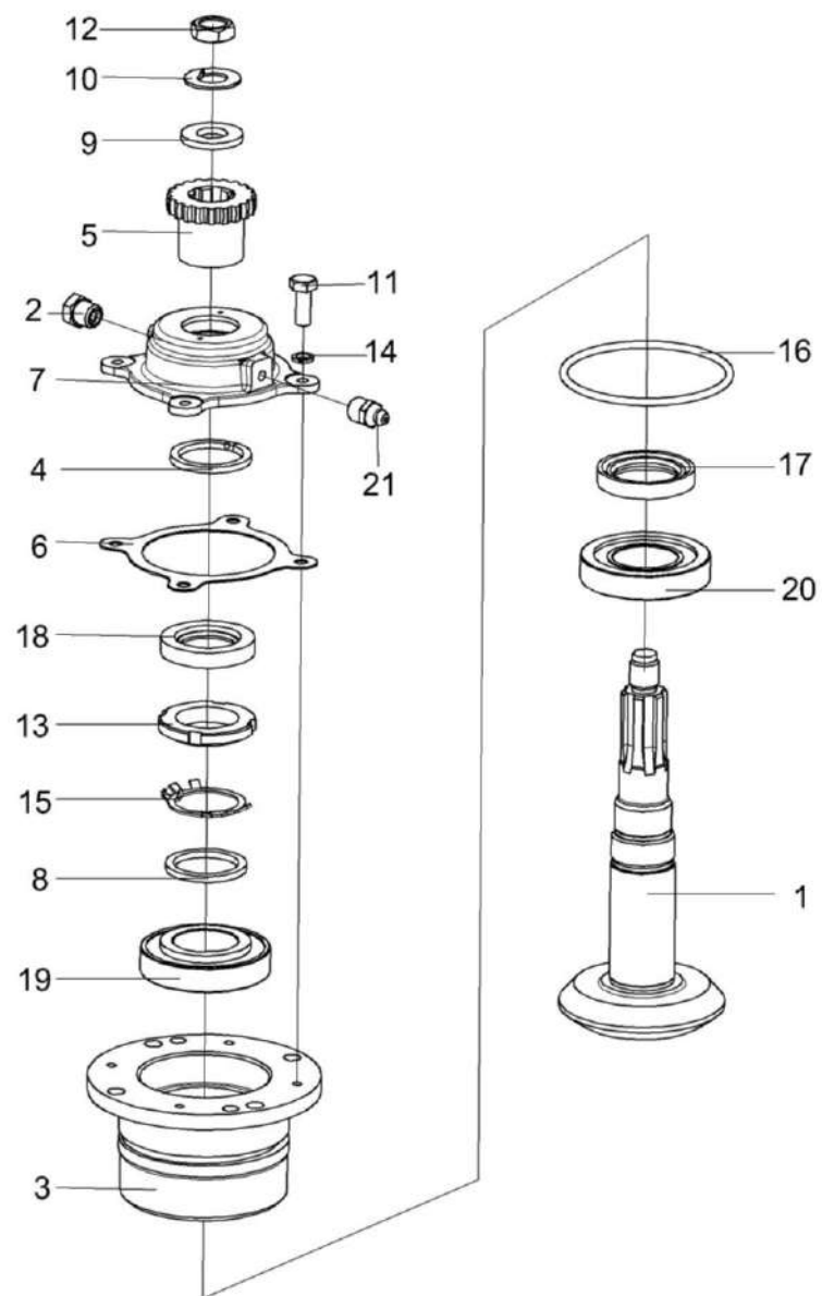
Рисунок 90 – Стакан КЗК-12-0209020
