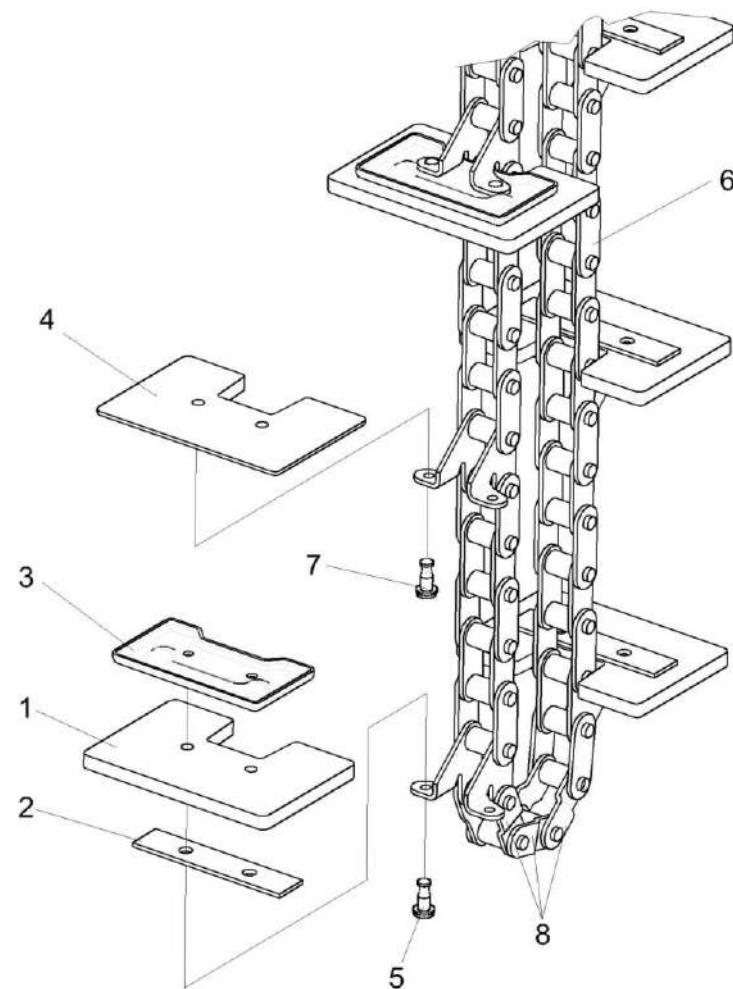
Рисунок 67 – Цепь элеватора КЗР 0208080Г
