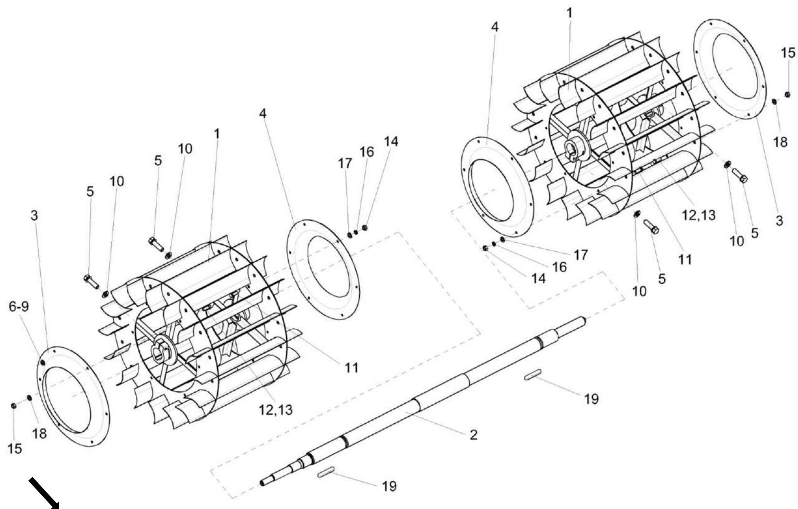
Рисунок 26 – Крылач КЗК 0217010В
