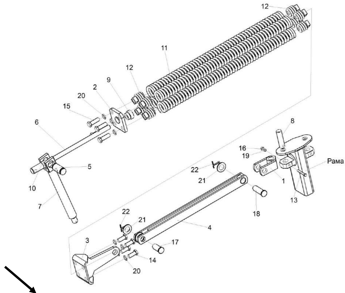
Рисунок 5 – Вывешивание боковой секции (правая) (изображено) Рисунок 6 – Вывешивание боковой секции (левая) (зеркальное отражение)
