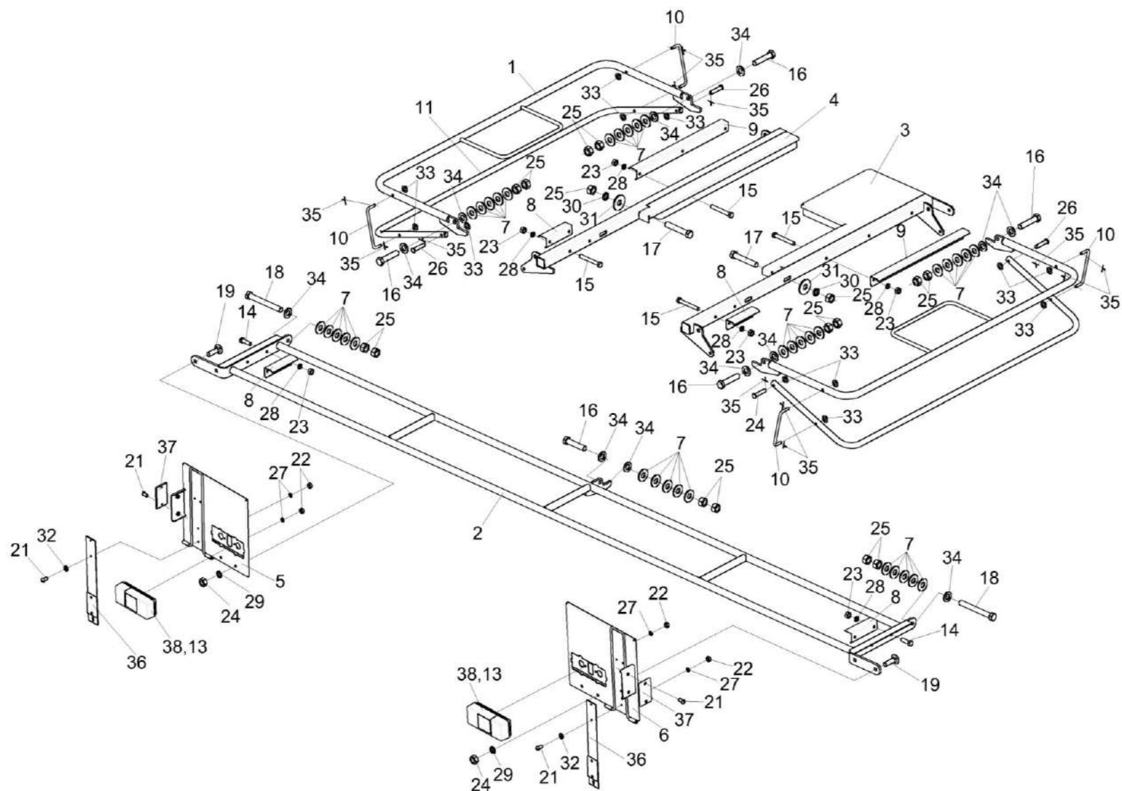
Рисунок 35 – Установка рамок, опор и дуг центральной секции
