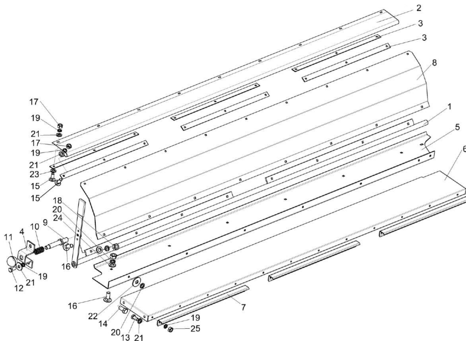
Рисунок 20 – Дека КПР-1-9200416 и рычаг КПР-1-9210000 (правая секция) (изображено) Рисунок 21 – Дека КПР-1-9200416 и рычаг КПР-1-9210000-01 (левая секция) (зеркальное отражение)
