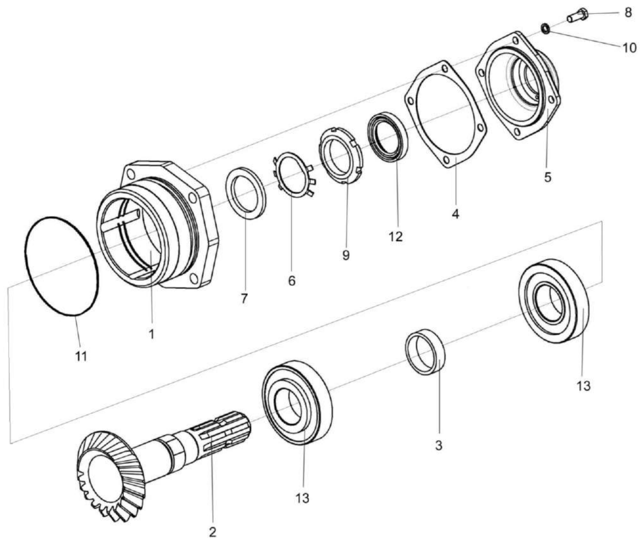
Рисунок 38 – Стакан КПР 9303010
