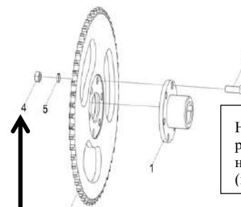
Рисунок 15 – Звездочка КЗК-1420-1527290
