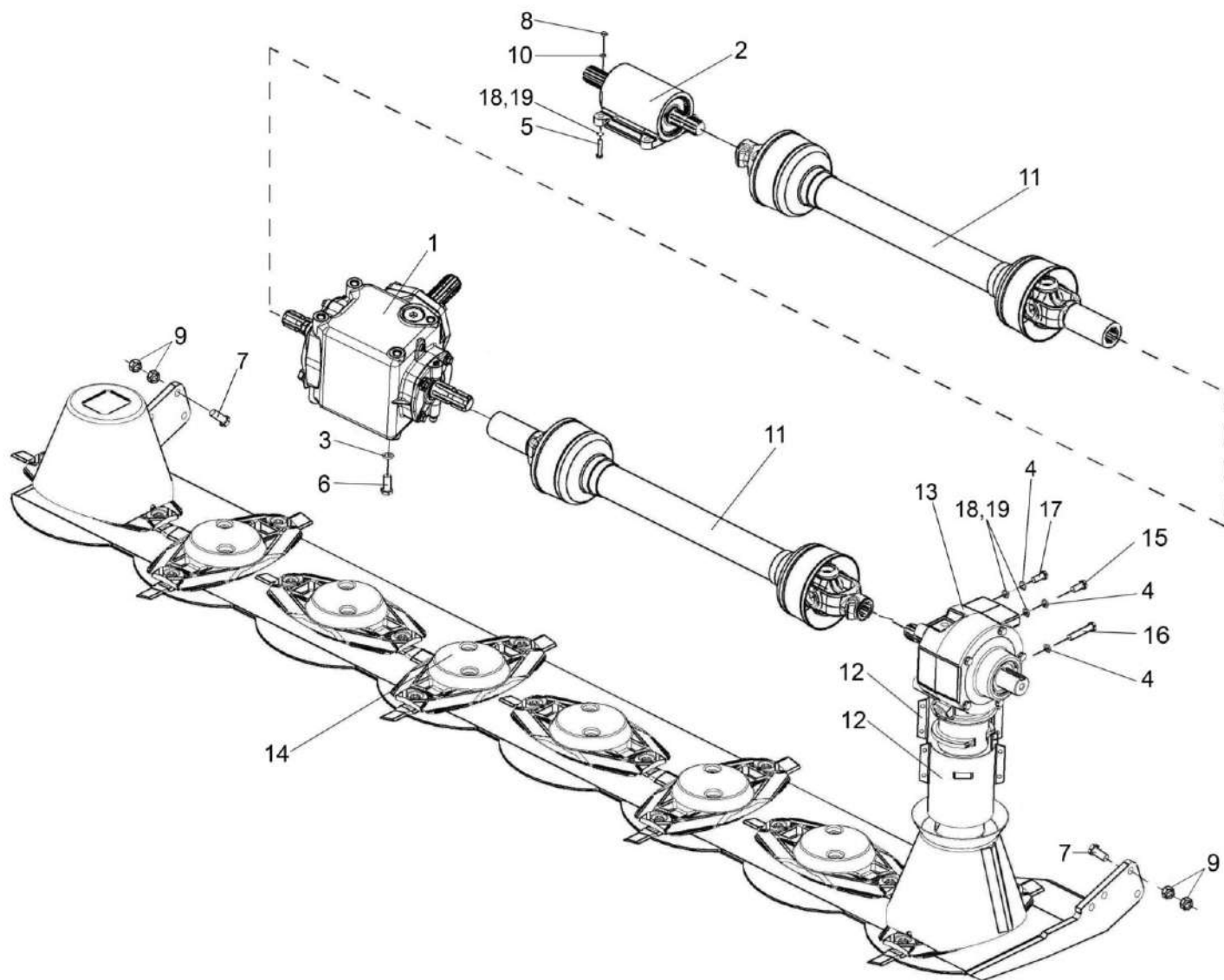
Рисунок 36 – Привод режущего аппарата центральной секции
