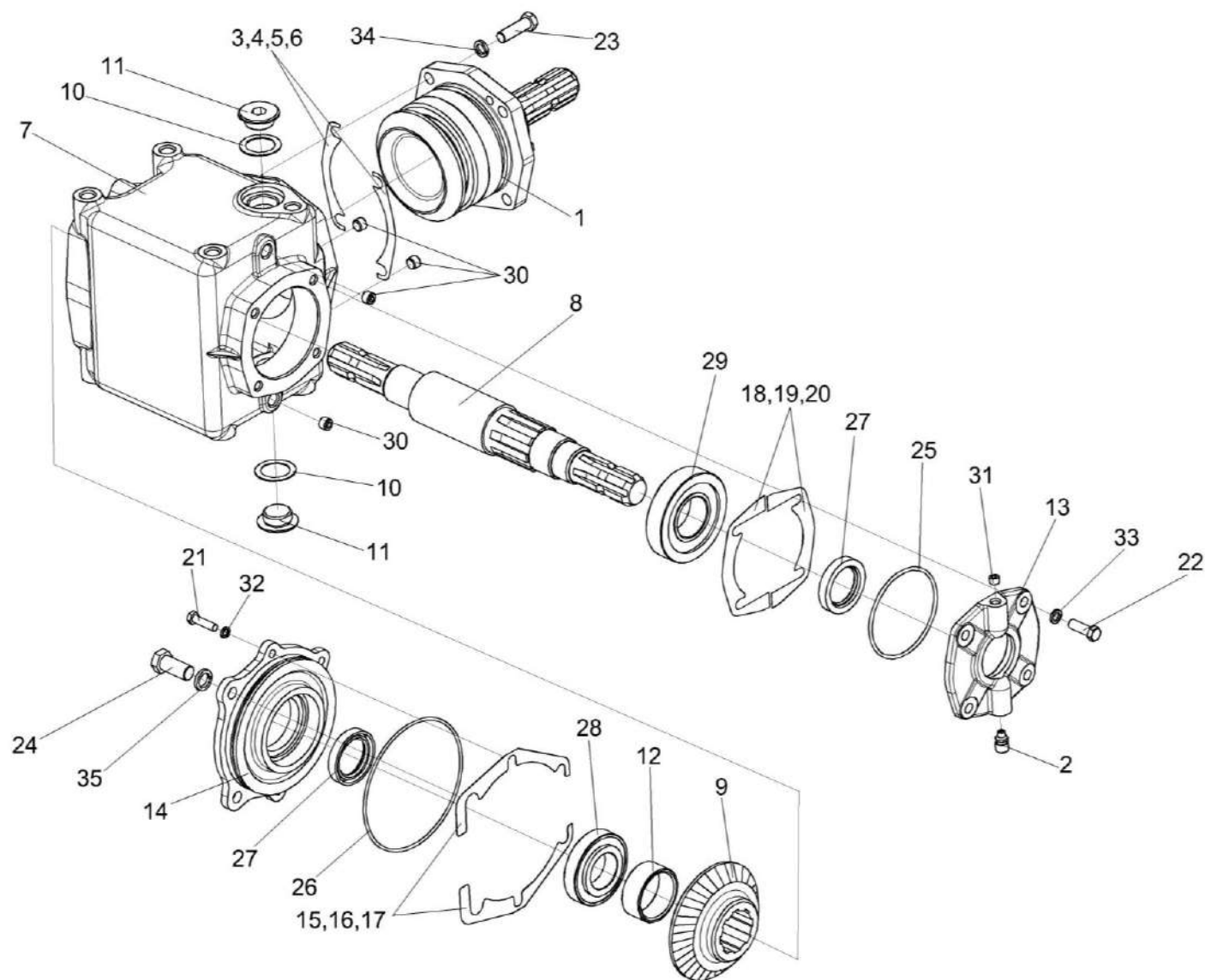
Рисунок 37 – Редуктор КПР 9303100
