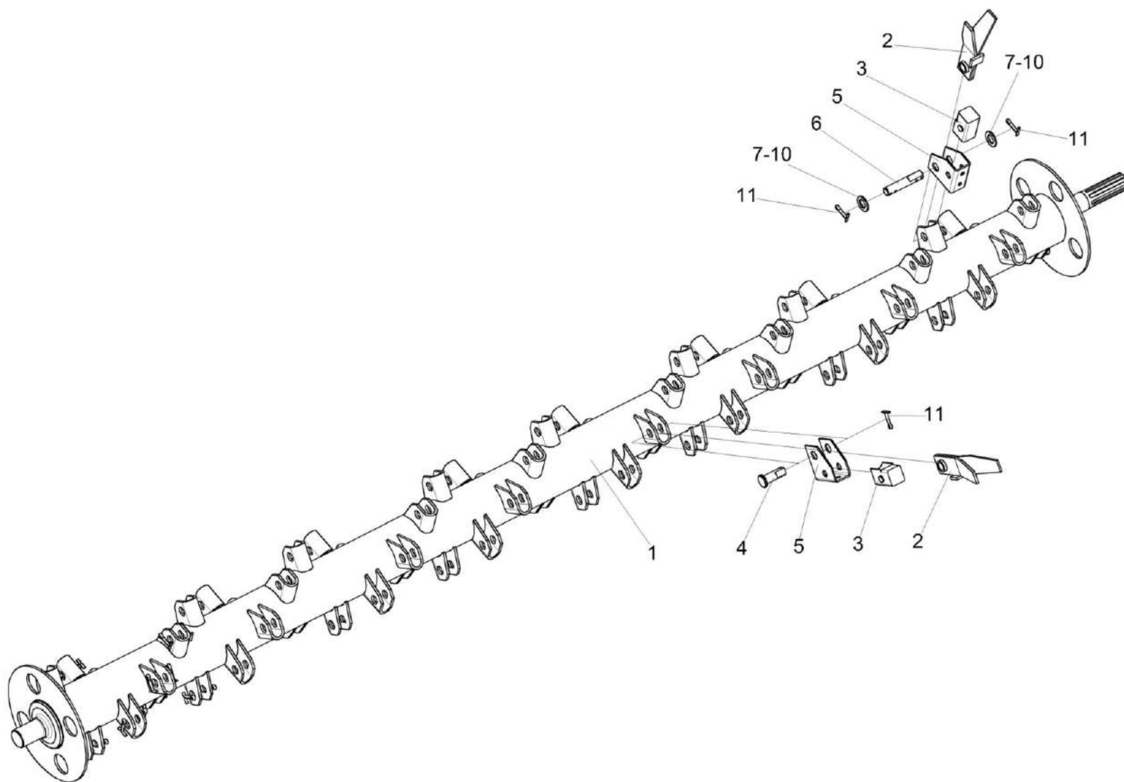
Рисунок 24 – Устройство бильное КПР 9202000Г (изображено)
