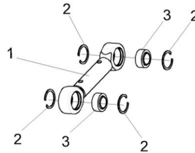
Рисунок 34 – Тяга КПР-9Т-9400110Э1
