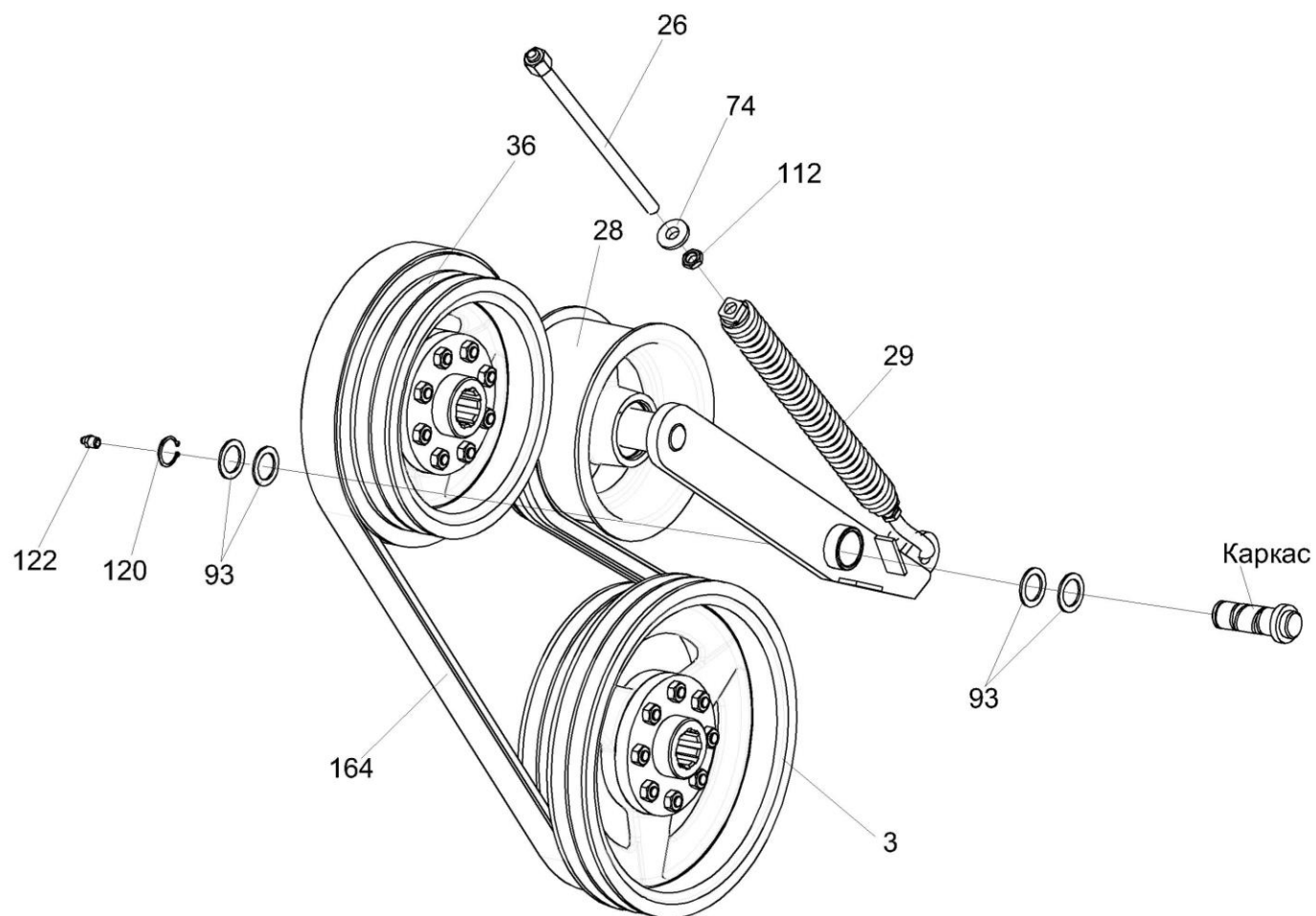
Рисунок 11 – Навеска передняя КПР 9500000А (установка устройства натяжного КПР 9206000А-01)
