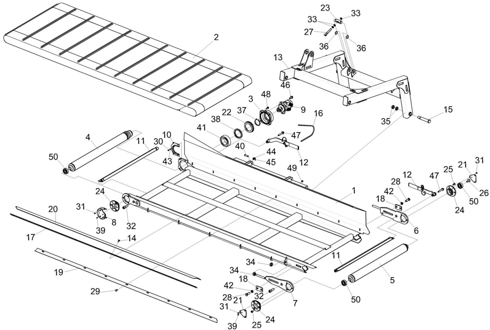
Рисунок 38 – Транспортер КПР-9Т-9600000Э1 и КПР-9Т-9600000Э1-01
