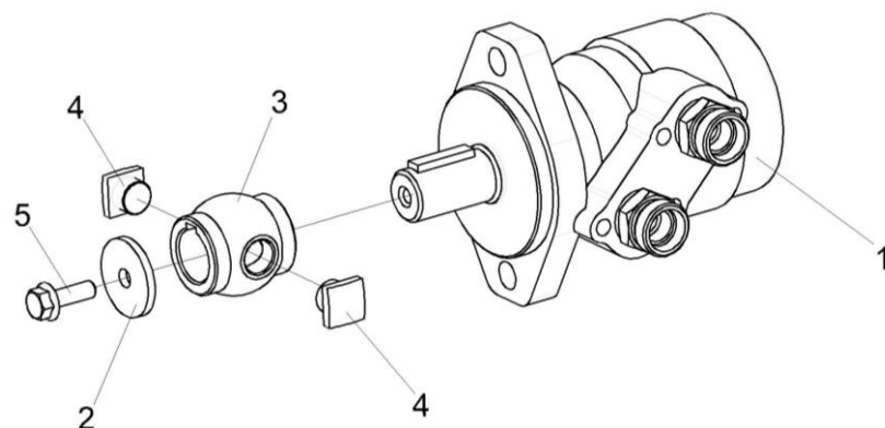
Рисунок 40 – Привод транспортера КПР-9Т-9600200Э1
