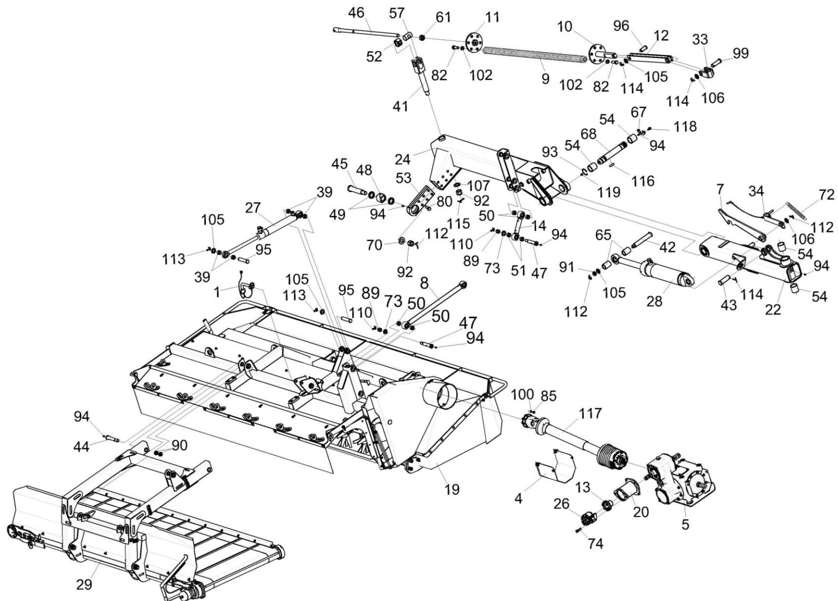
Рисунок 21 – Навеска задняя КПР-9Т-9400000Э1 (лист 1)
