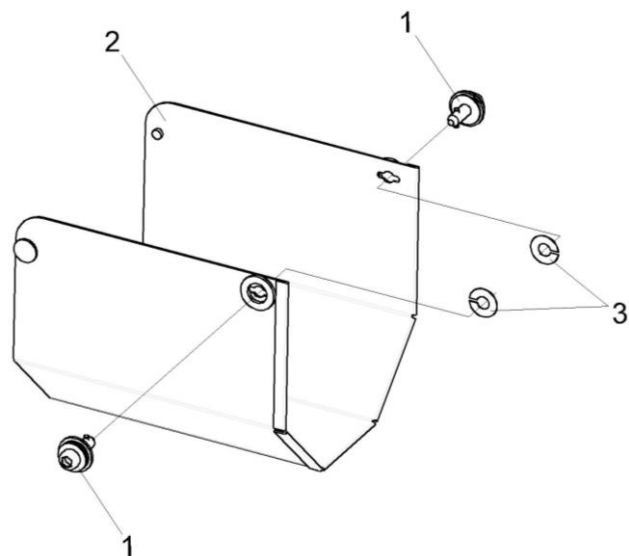
Рисунок 25 – Щиток КПР-1-9400040
