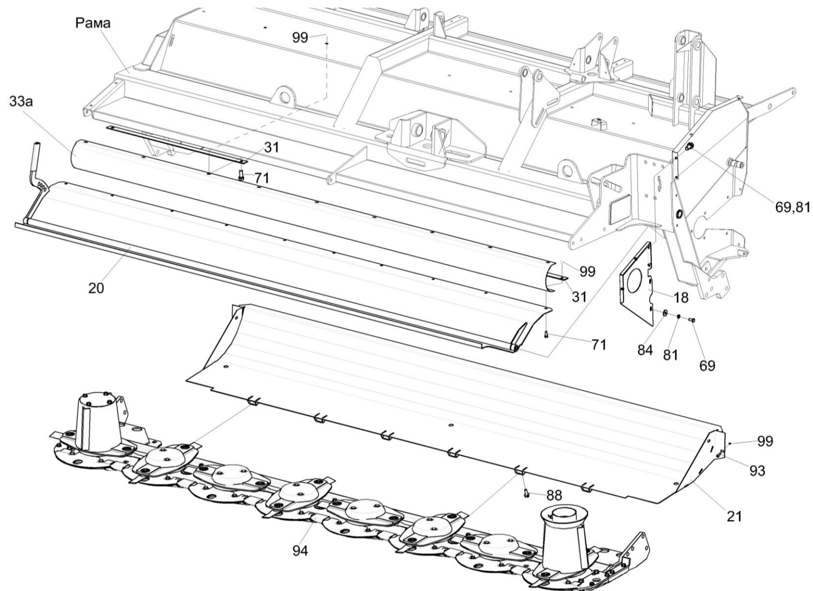
Рисунок 52 - КПР-9Т-9402000-Секция боковая (установка деки и поддона, рычагов)(изображено) и КПР-9Т-9402000-01-Секция боковая (установка деки и поддона, рычагов)(зеркальное отражение)
