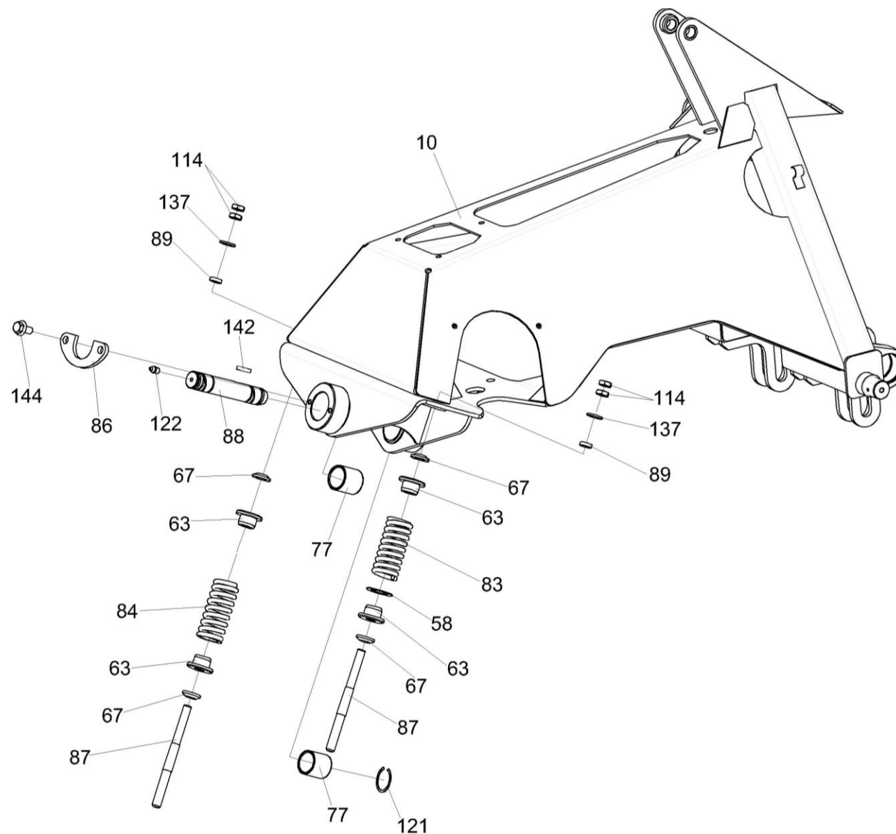
Рисунок 6 – Навеска передняя КПР 9500000А (установка рамы КПР-1-9301100А)
