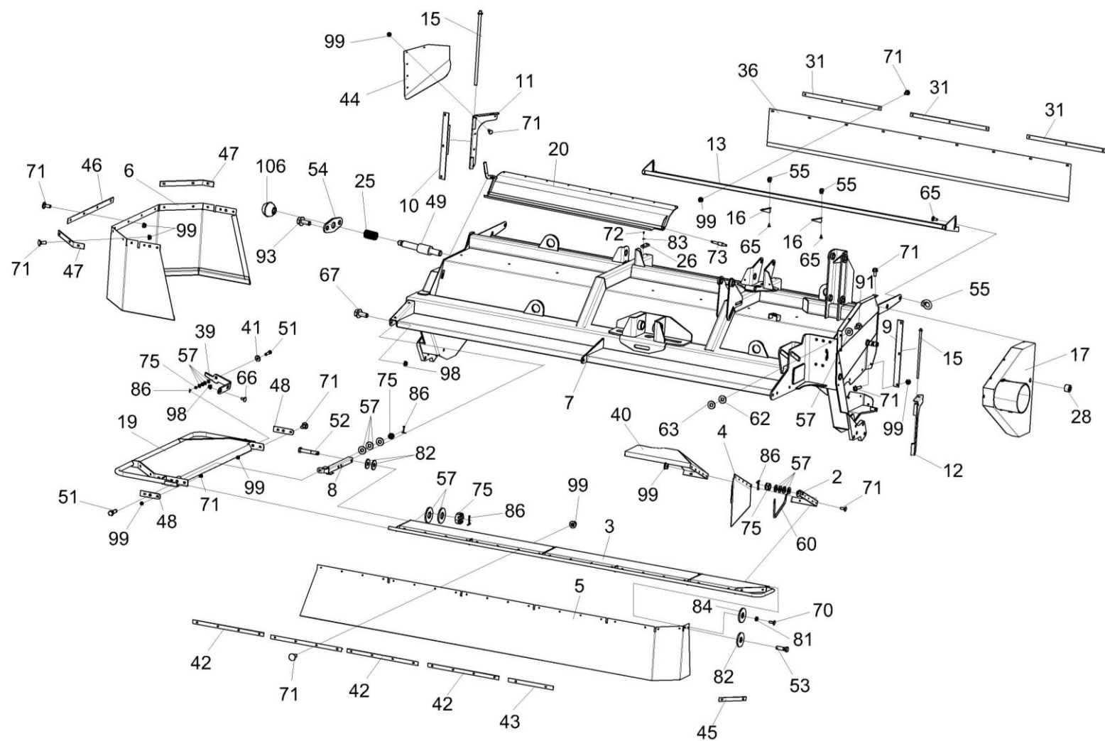
Рисунок 43 – Секция боковая КПР-9Т-9402000Э1 (установка прижимов, щитков и половов)
