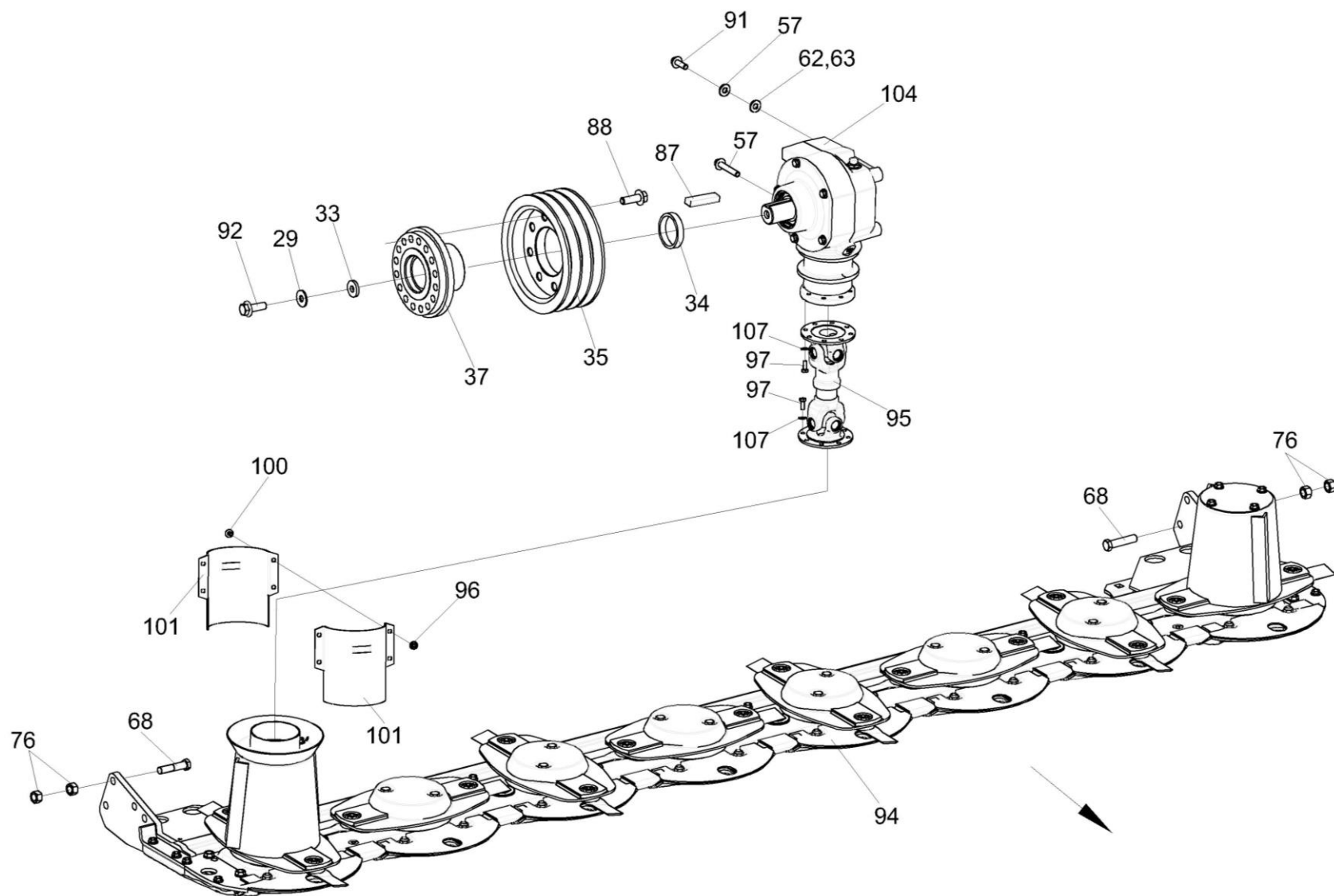
Рисунок 50 – Секция боковая КПР-9Т-9402000Э1-01 (привод режущего аппарата левой секции)
