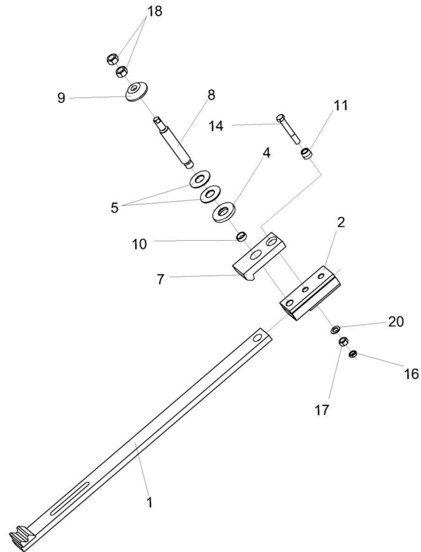
Рисунок 41 – Устройство предохранительное КПР9133000
