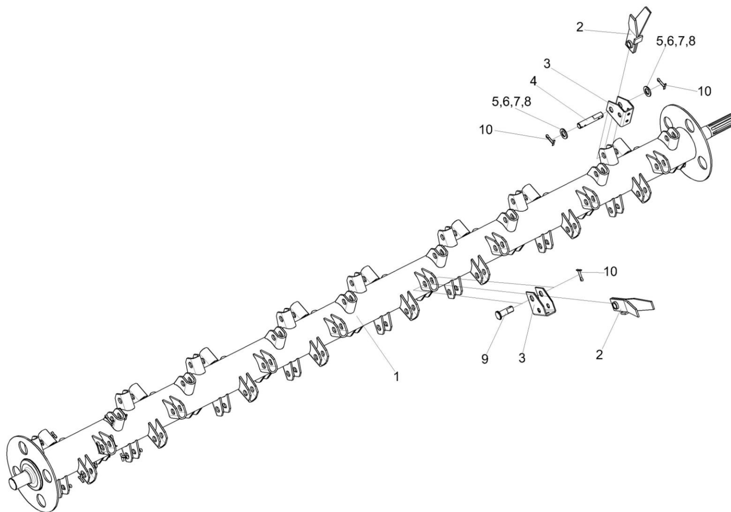
Рисунок 55 – Устройство бильное КПР 9202000Г (изображено) и КПР 9202000Г-01 (зеркальное отражение)
