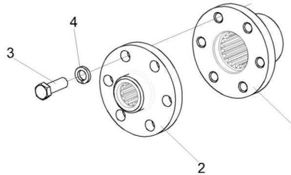
Рисунок 33 – Муфта КПР-9Т-9400100Э1
