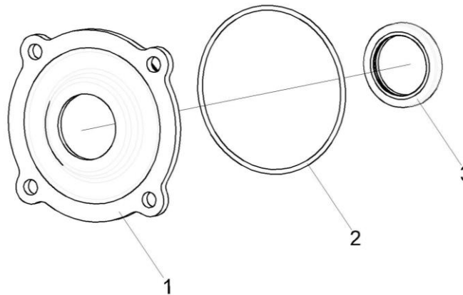
Рисунок 29 – Крышка КПР-1-9403110
