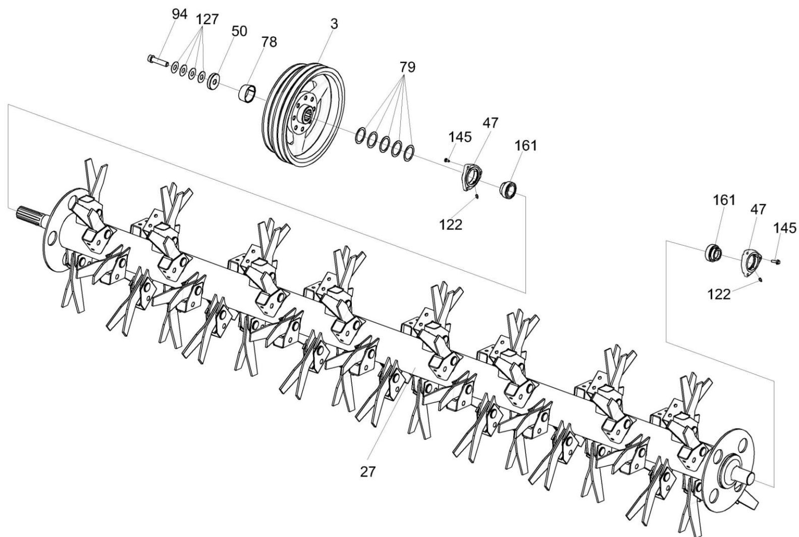
Рисунок 10 – Навеска передняя КПР 9500000А (установка бильного устройства центральной секции)
