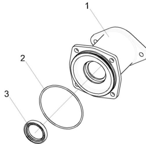
Рисунок 36 – Фланец КПР-9Т-9403010Э1
