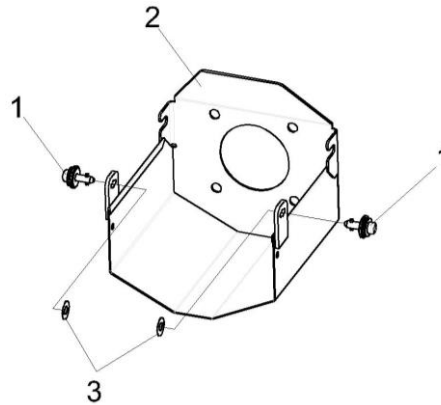
Рисунок 35 – Кожух КПР-9Т-9400140Э1
