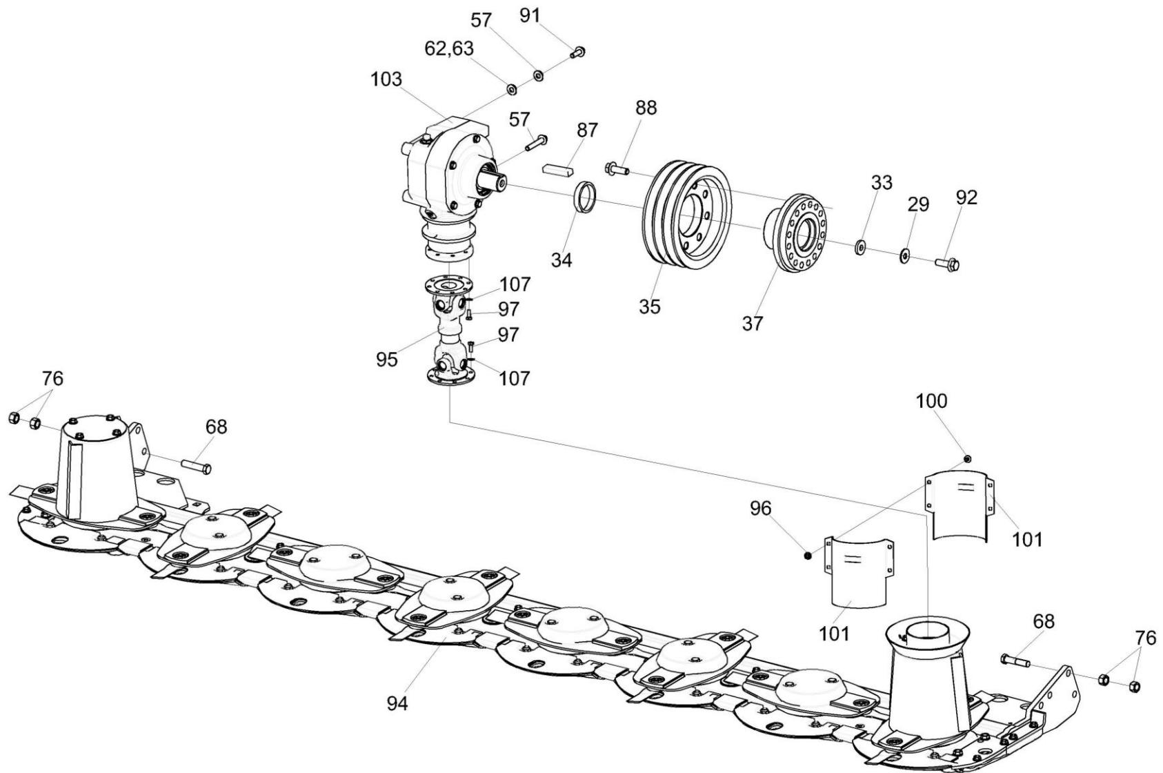
Рисунок 45 – Секция боковая КПР-9Т-9402000Э1 (привод режущего аппарата правой секции)
