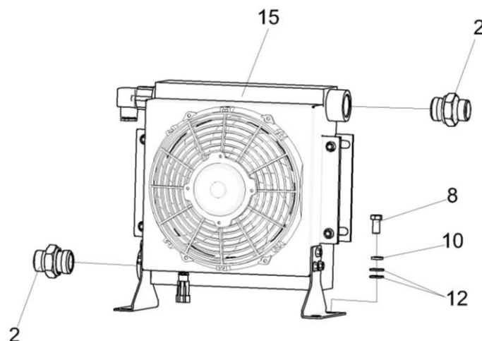
Рисунок 63 – Радиатор масляный КПР-9Т-9460490Э1
