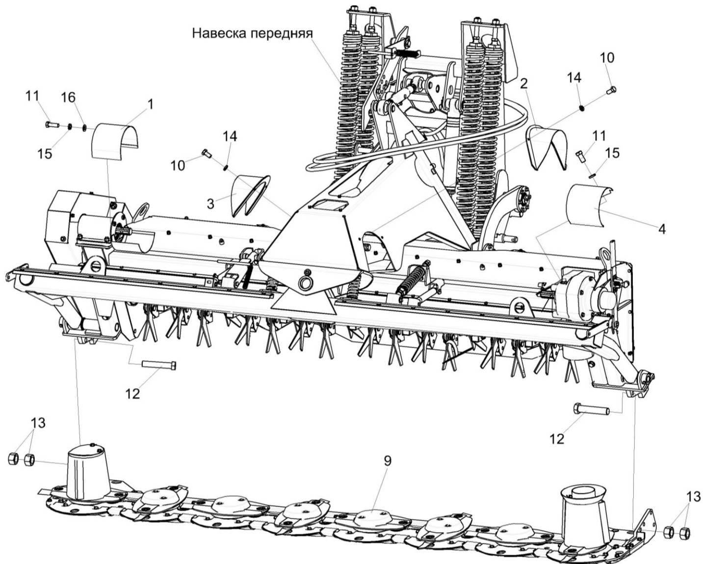
Рисунок 4 – Навеска передняя КПР 9500000А (установка режущего аппарата и кожухов)
