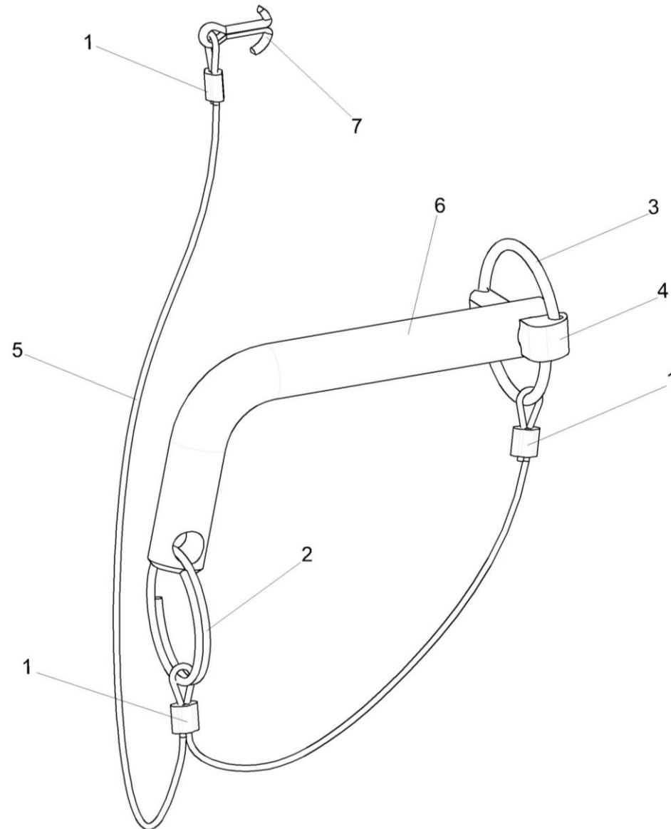
Рисунок 24 – Фиксатор КВП0102030
