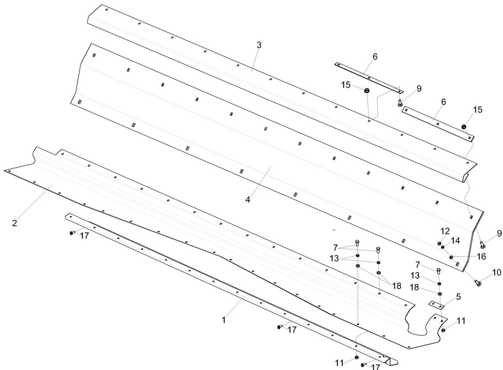
Рисунок 8 – Навеска передняя КПР 9500000А (установка деки и порога центральной секции)
