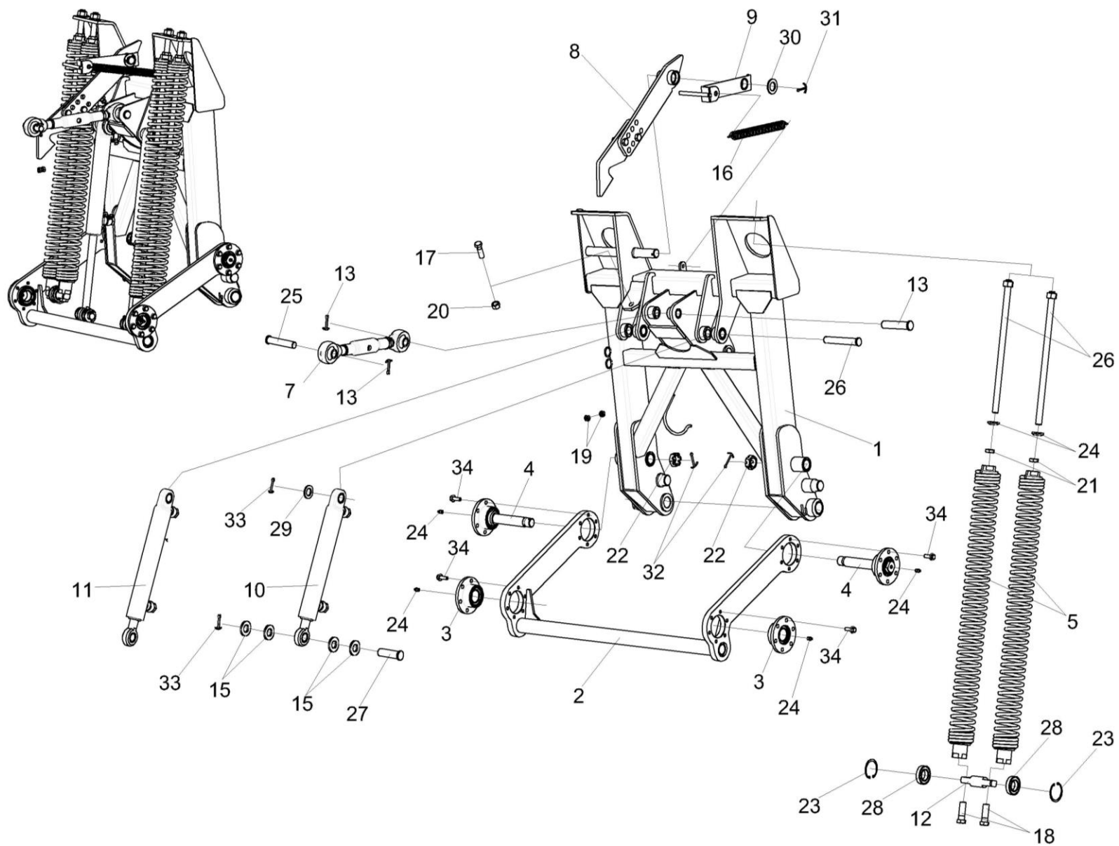
Рисунок 16 – Установка рамки переходной КПР-1-9300010А
