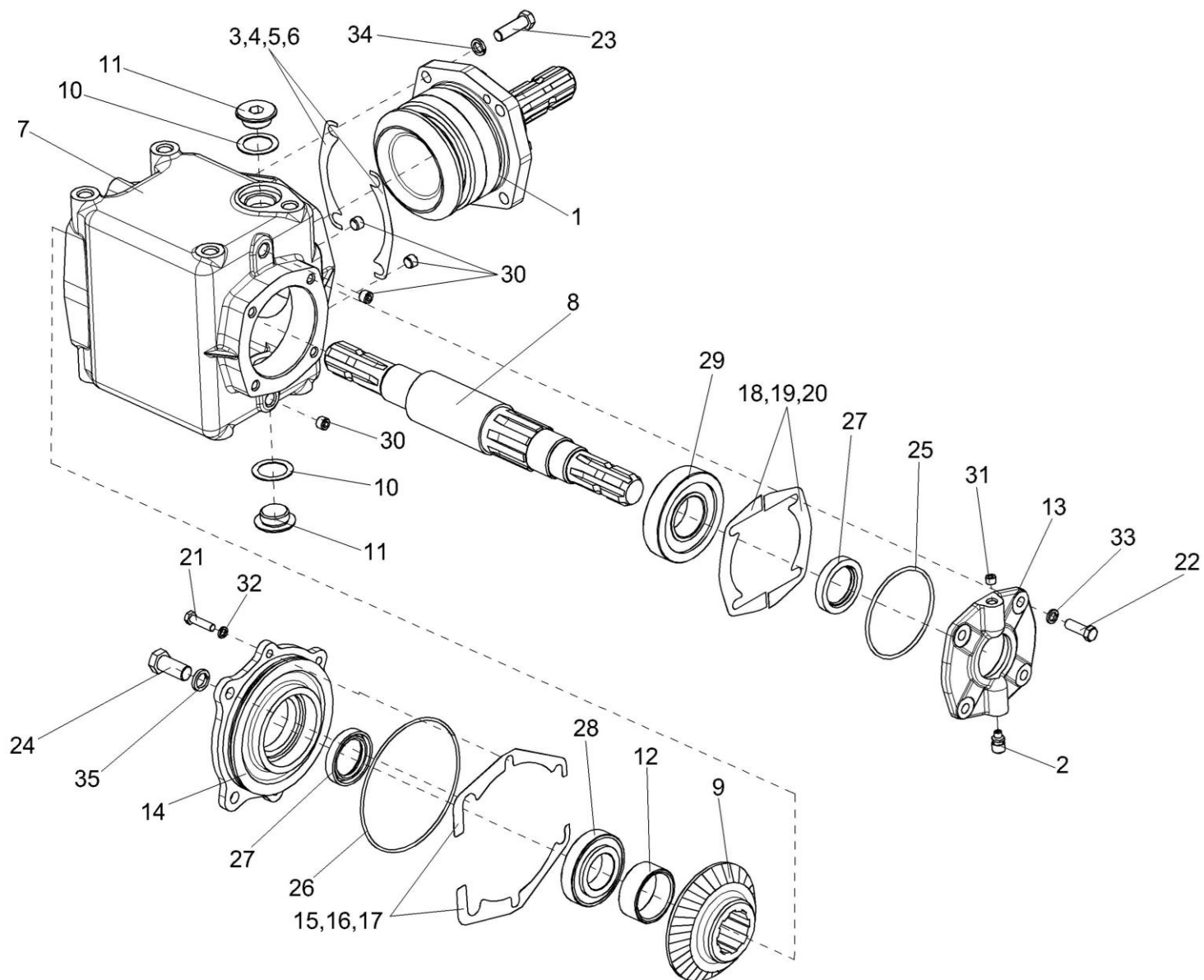
Рисунок 17 – Редуктор КПР 9303100-01
