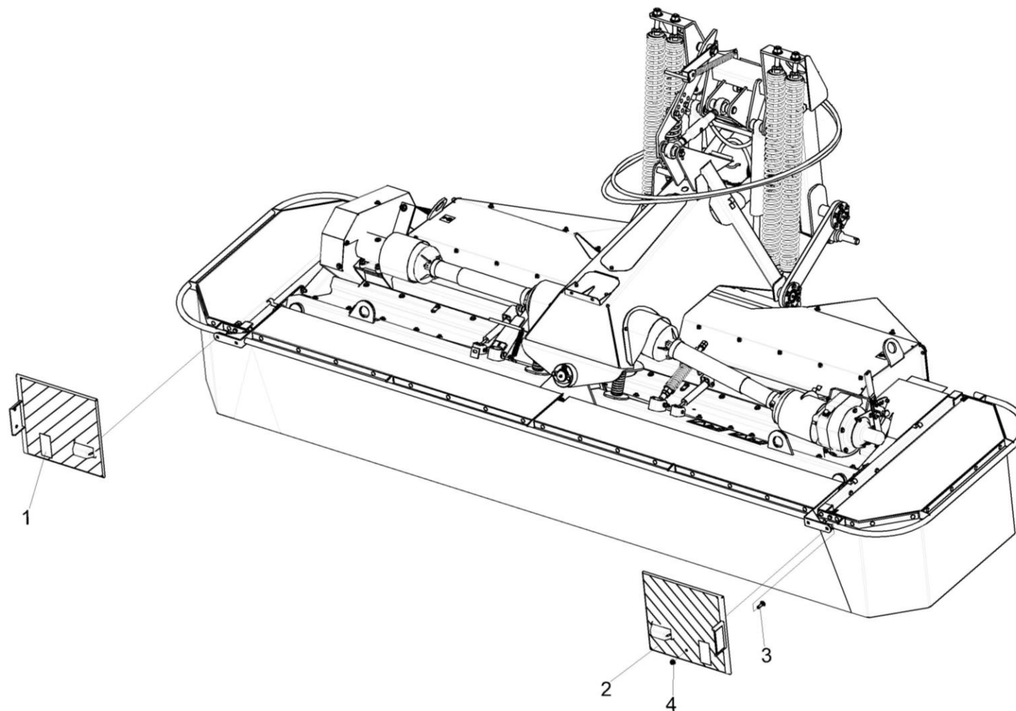
Рисунок 68 – Установка щитков КПР-9Т-9000050Э1
