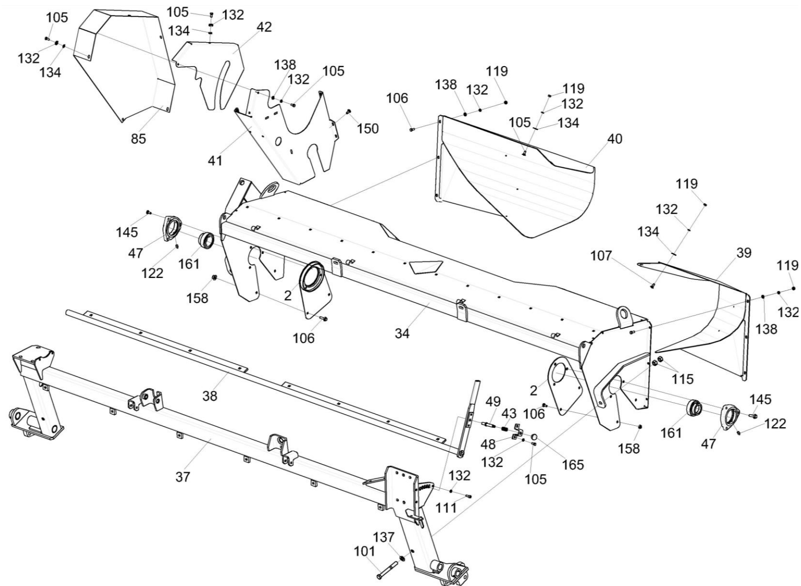
Рисунок 7 – Навеска передняя КПР 9500000А (установка каркаса, рамы и щитков)
