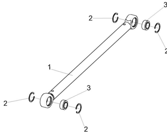
Рисунок 31 – Тяга КПР-9Т-9400020Э1
