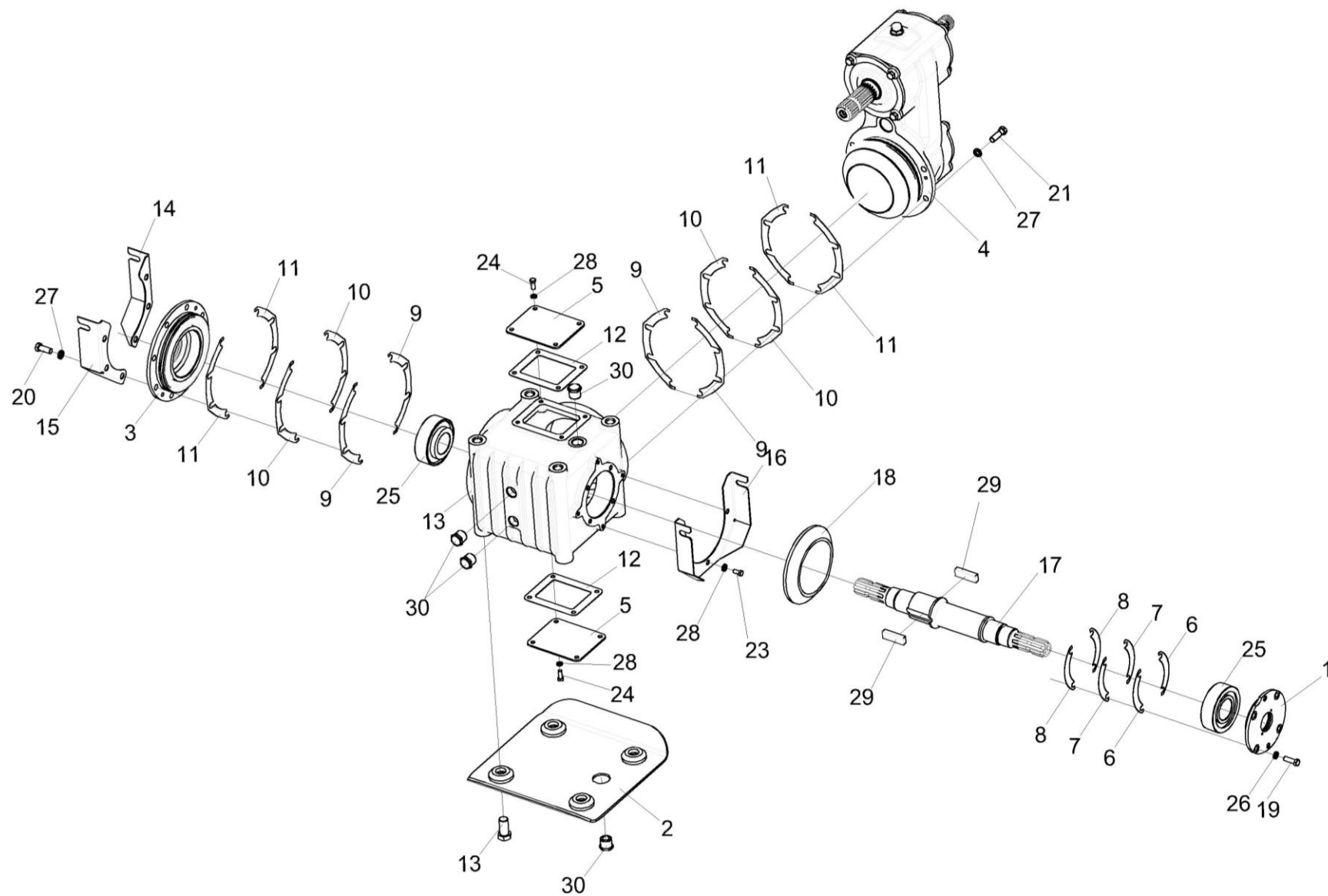
Рисунок 26 – Редуктор КПР-1-9403000-02
