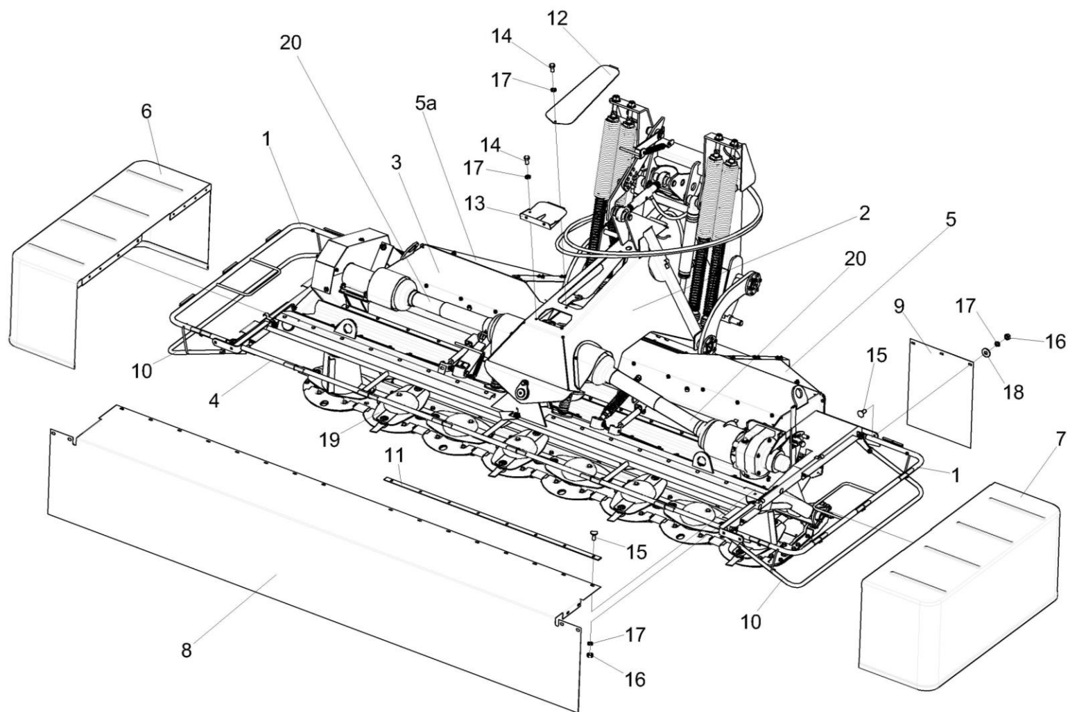
Рисунок 2 – Навеска передняя КПР 9500000А (установка полов, крышки и кронштейна)
