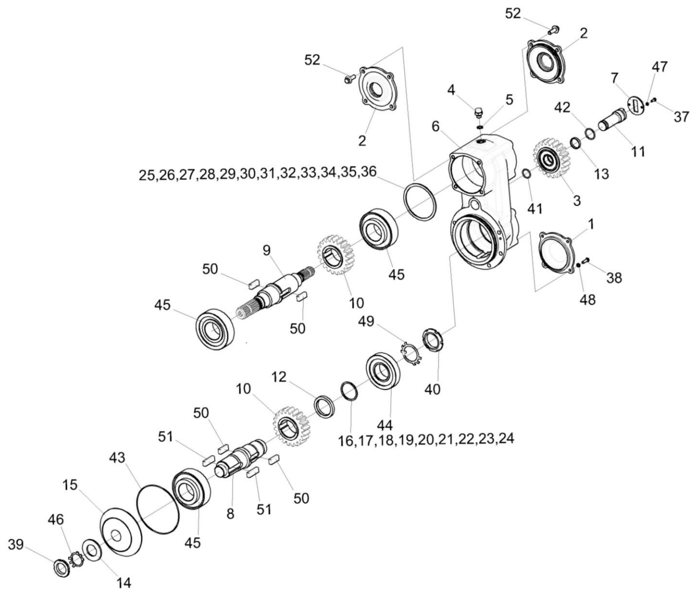
Рисунок 27 – Редуктор КПР-1-9403100
