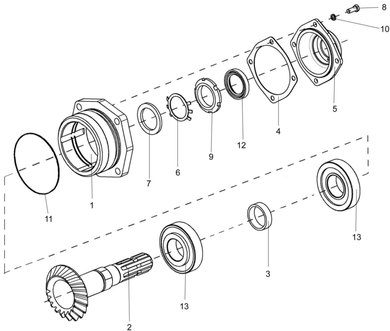
Рисунок 18 – Стакан КПР 9303010
