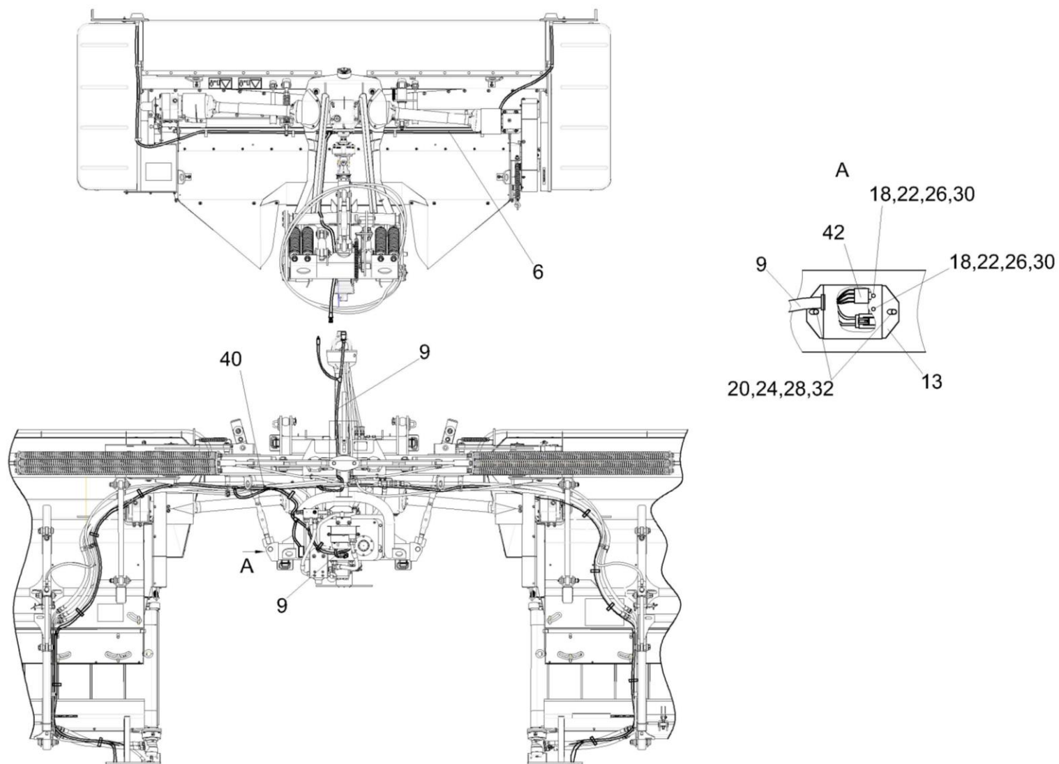
Рисунок 70 – Установка электрооборудования КПР-9Т-9721000Э1
