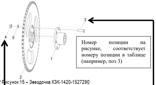
Рисунок 15 – Звездочка КЗК-1420-1527290
