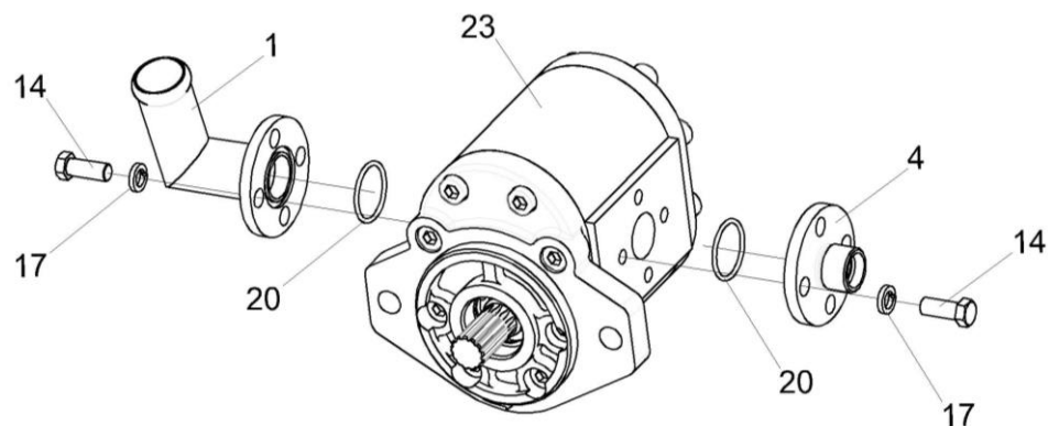
Рисунок 37 – Гидронасос шестеренный КПР-9Т-9460100Э1
