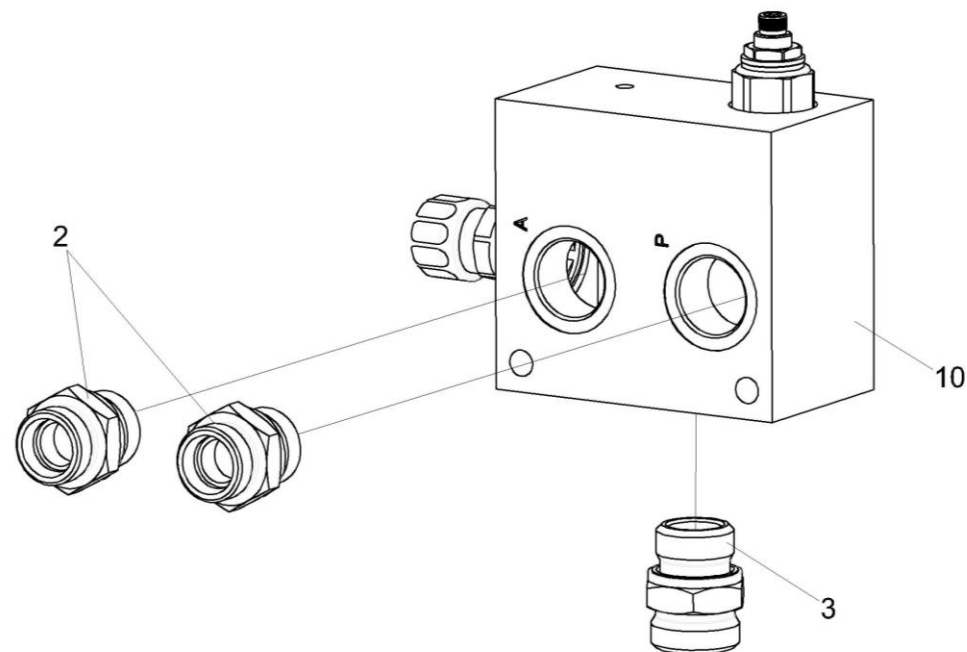
Рисунок 66 – Регулятор расхода КПР-9Т-9460300Э1
