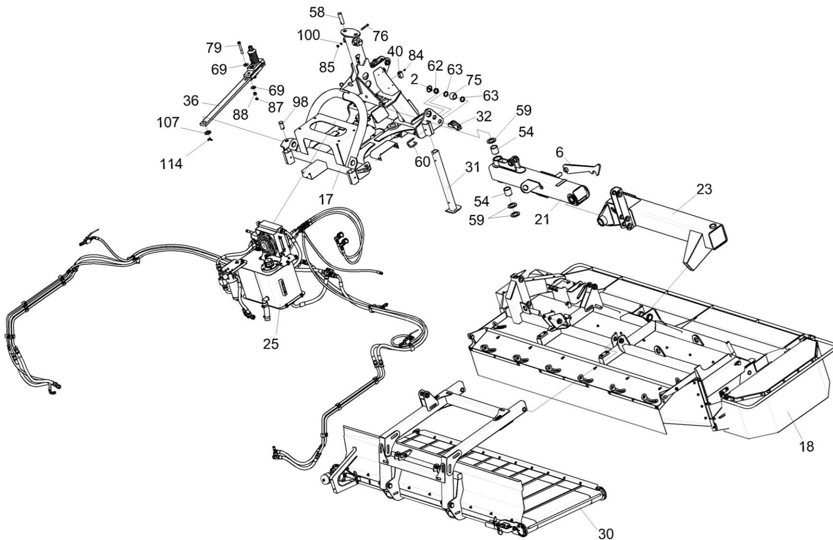
Рисунок 22 – Навеска задняя КПР-9Т-9400000Э1 (лист 2)
