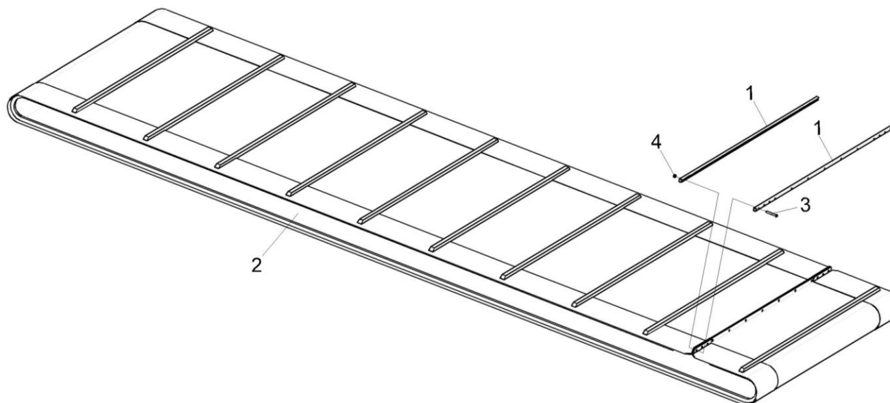
Рисунок 39 – Лента транспортерная КПР-9Т-9600060Э1
