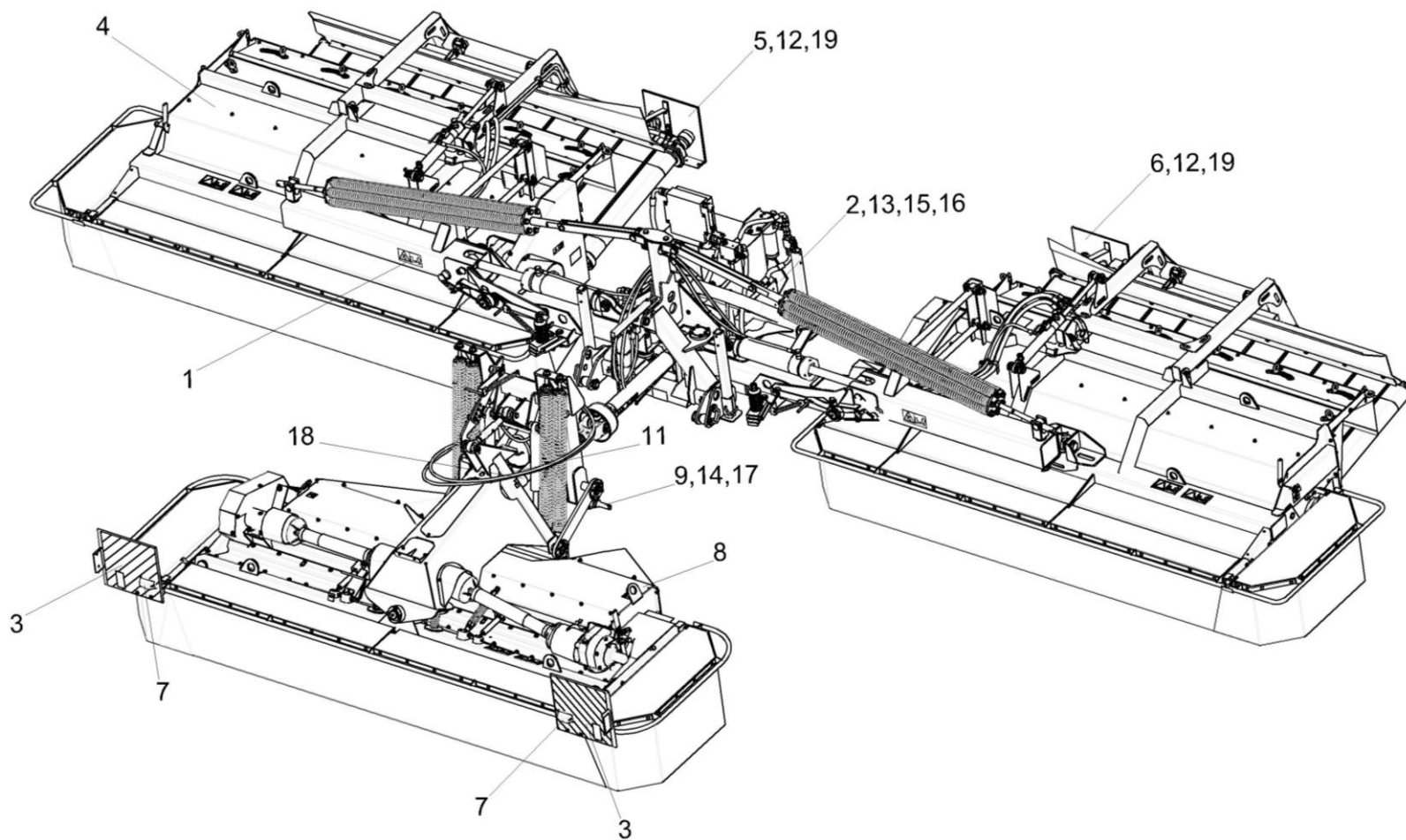
Рисунок 1 – Косилка-плющилка ротационная трехсекционная навесная КПР-9Т (КПР-9Т-9000000Э1)
