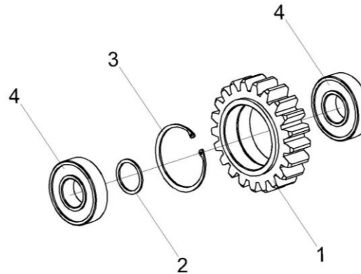
Рисунок 30 – Колесо зубчатое КПР-1-9403120
