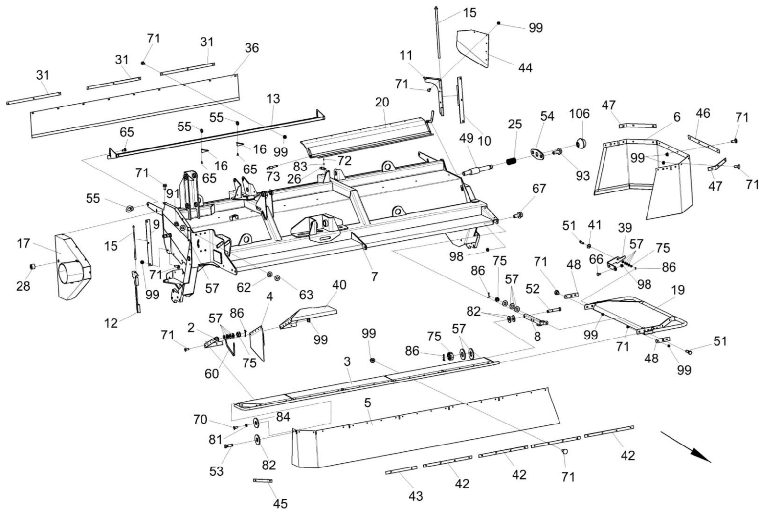
Рисунок 48 – Секция боковая КПР-9Т-9402000Э1-01 (установка прижимов, щитков и полов)
