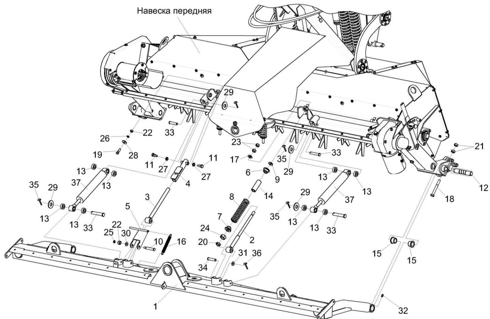
Рисунок 5 – Навеска передняя КПР 9500000А (установка коромысла КПР 9504000)
