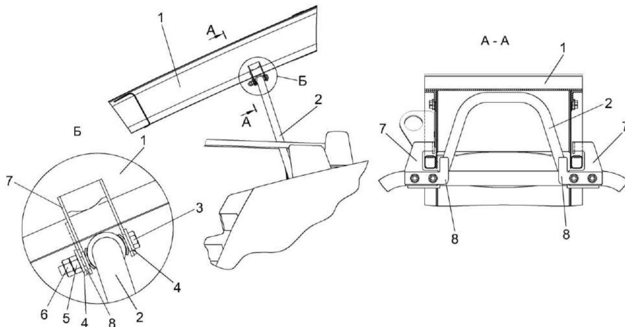
Рисунок 2.3 – Механизм фиксации силосопровода
