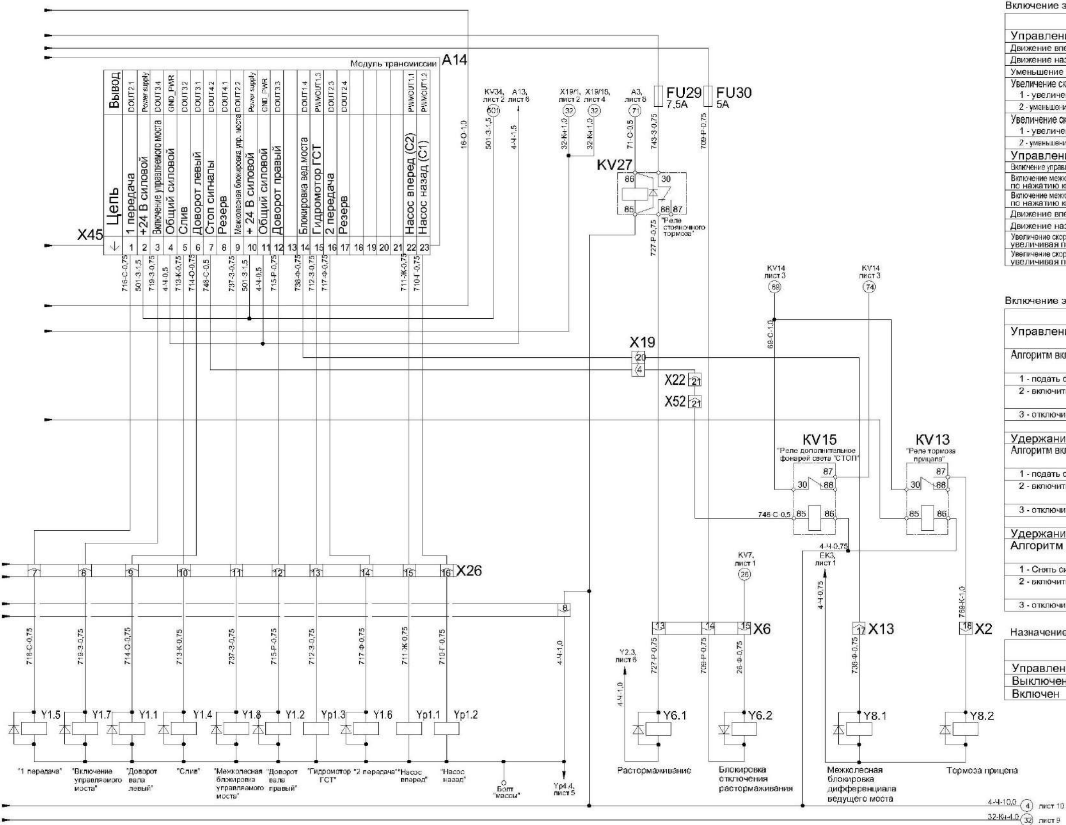
Рисунок Б.1 – Схема электрическая принципиальная комбайна (лист 76)
