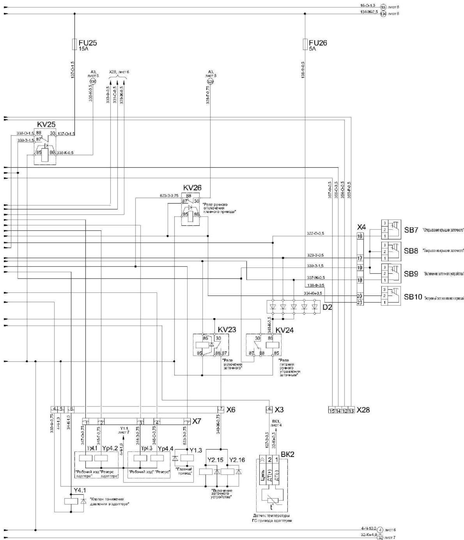
Рисунок Б.1 - Схема электрическая принципиальная комбайна (лист 56)
