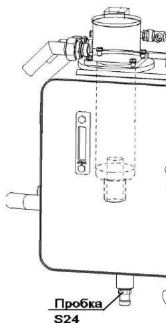
Рисунок 3.6 – Сливной штуцер
