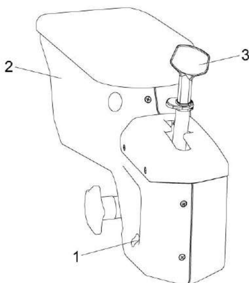
1 - болт регулировочный; 2 – корпус блока управления; 3 – рукоятка управления скоростью
