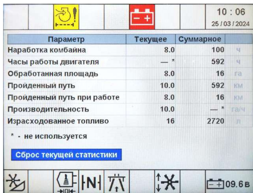
Рисунок К.18 – Вид окна «Статистика»
