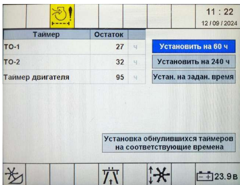
Рисунок К.19 – Вид окна «Интервалы ТО»
