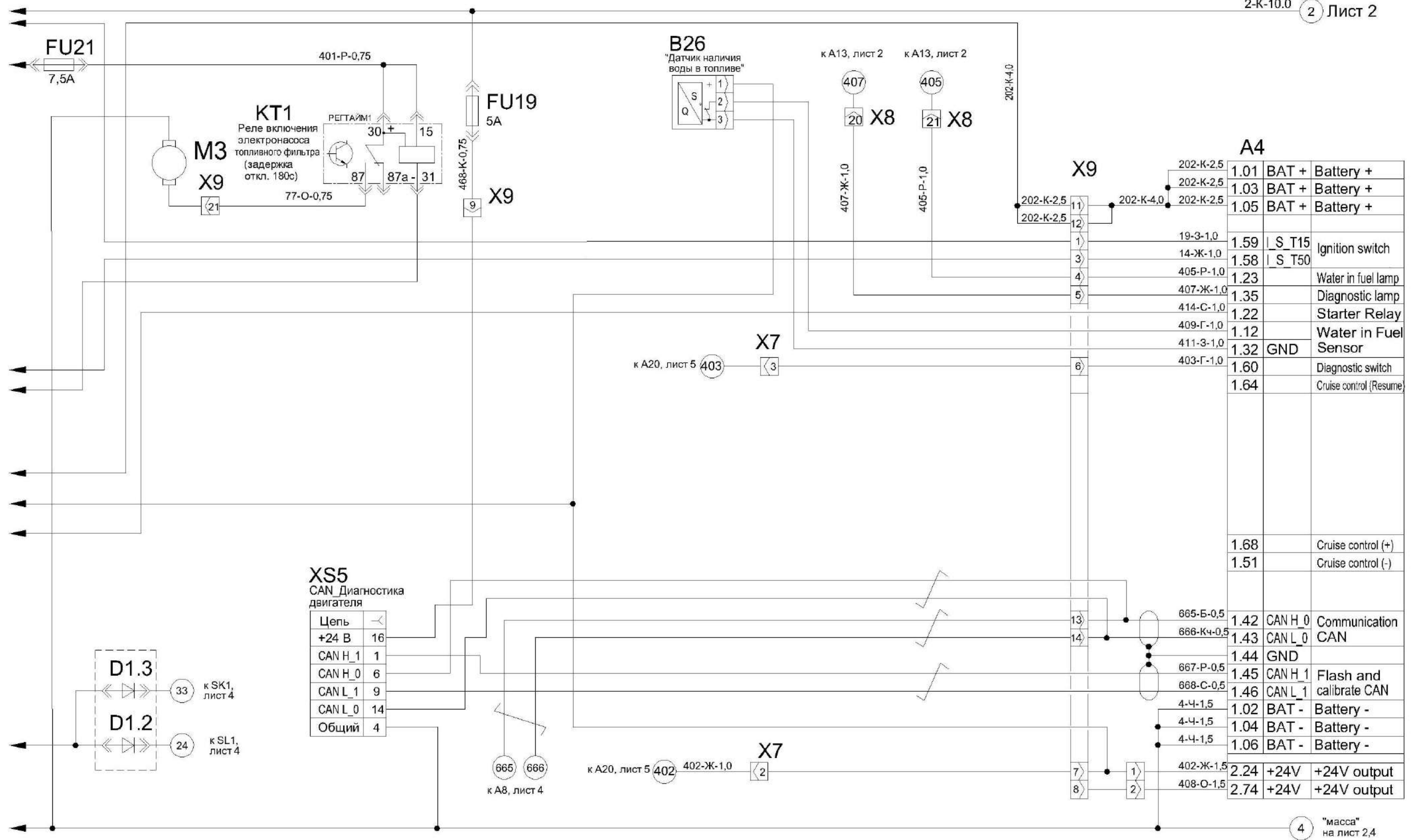
Рисунок Б.1 – Схема электрическая принципиальная косилки самоходной (лист 16)
