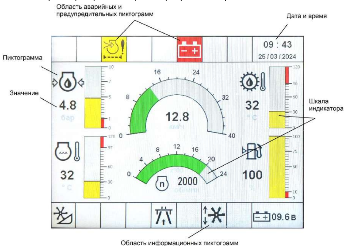
Рисунок К.2 – Экран «Дорога»
