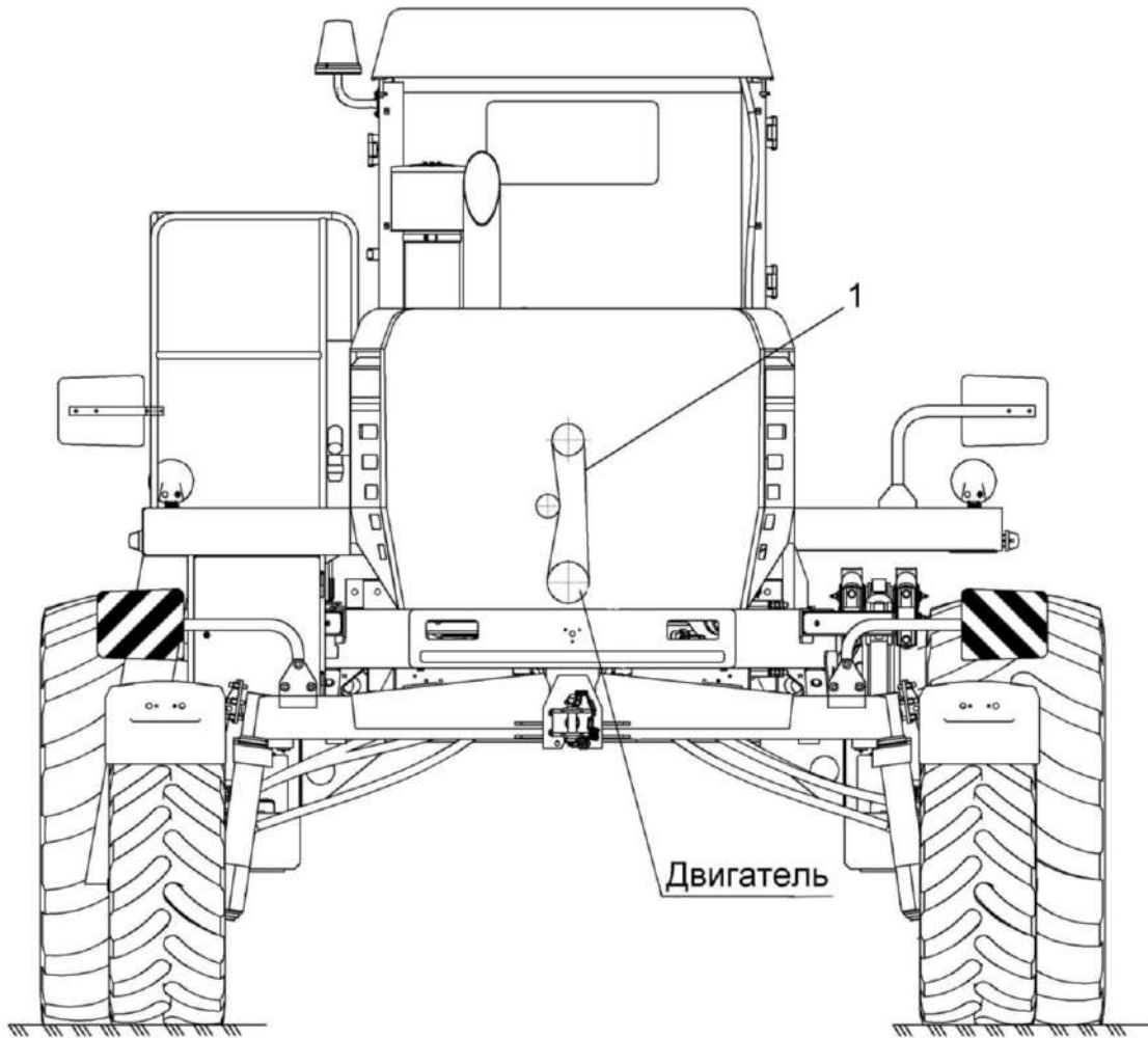
Рисунок – Схема приводов косилки
